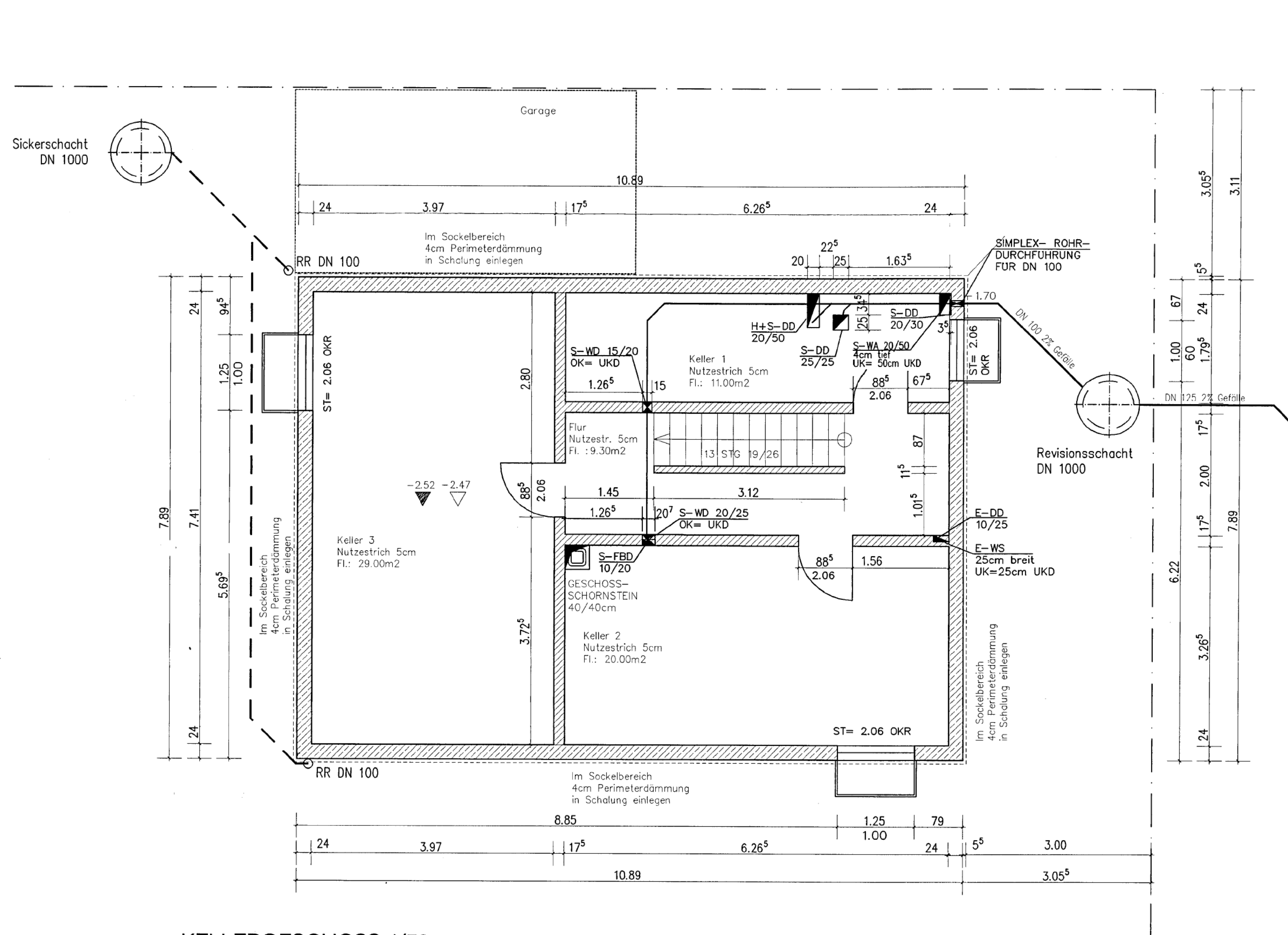
KELLERGESCHOSS 1/50
