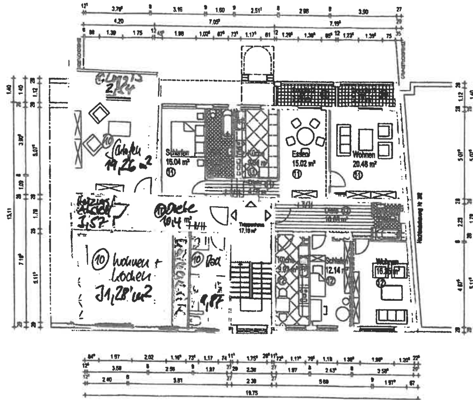
3. OBERGESCHOSS
