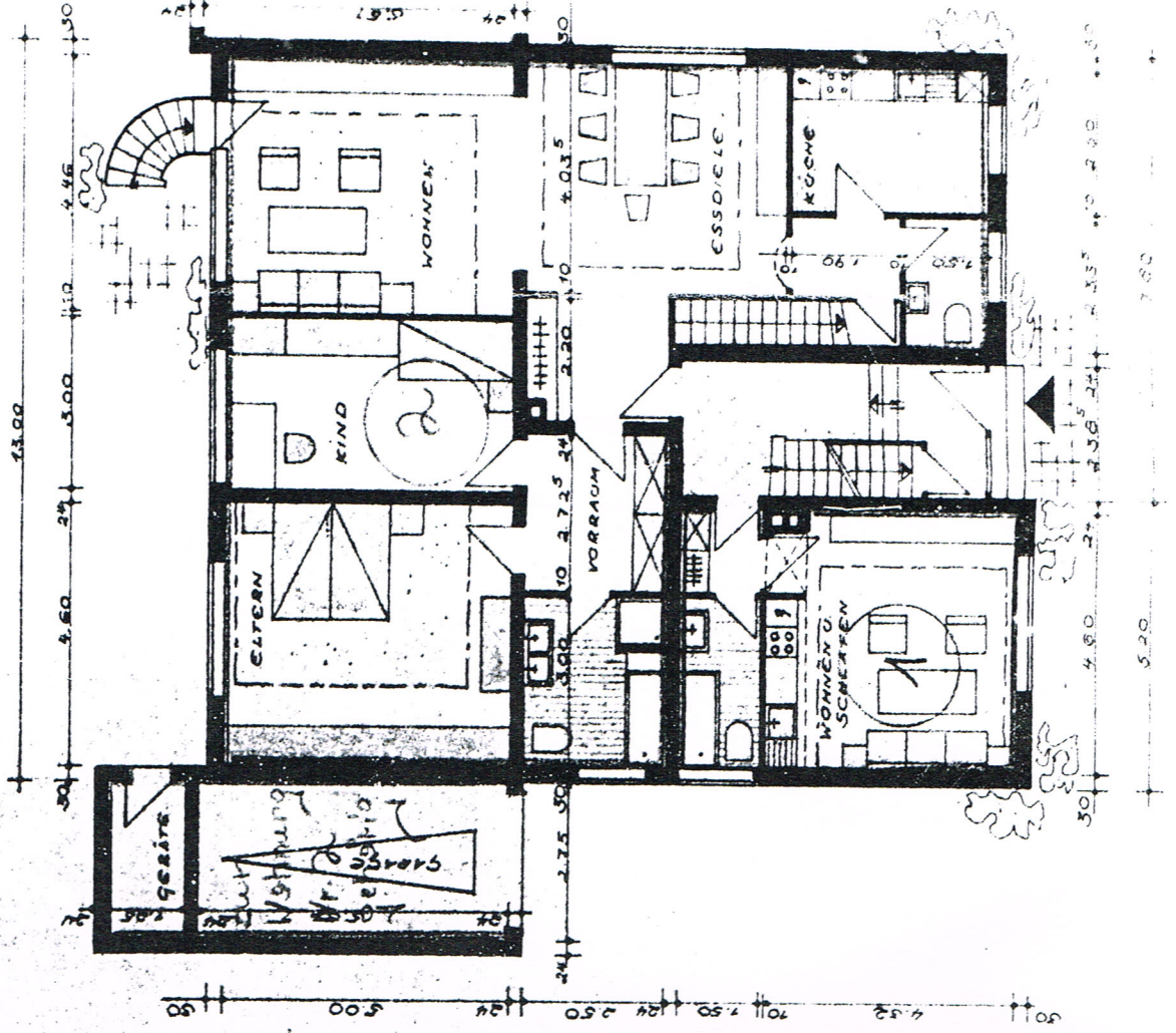
ERDGESCHOSS
