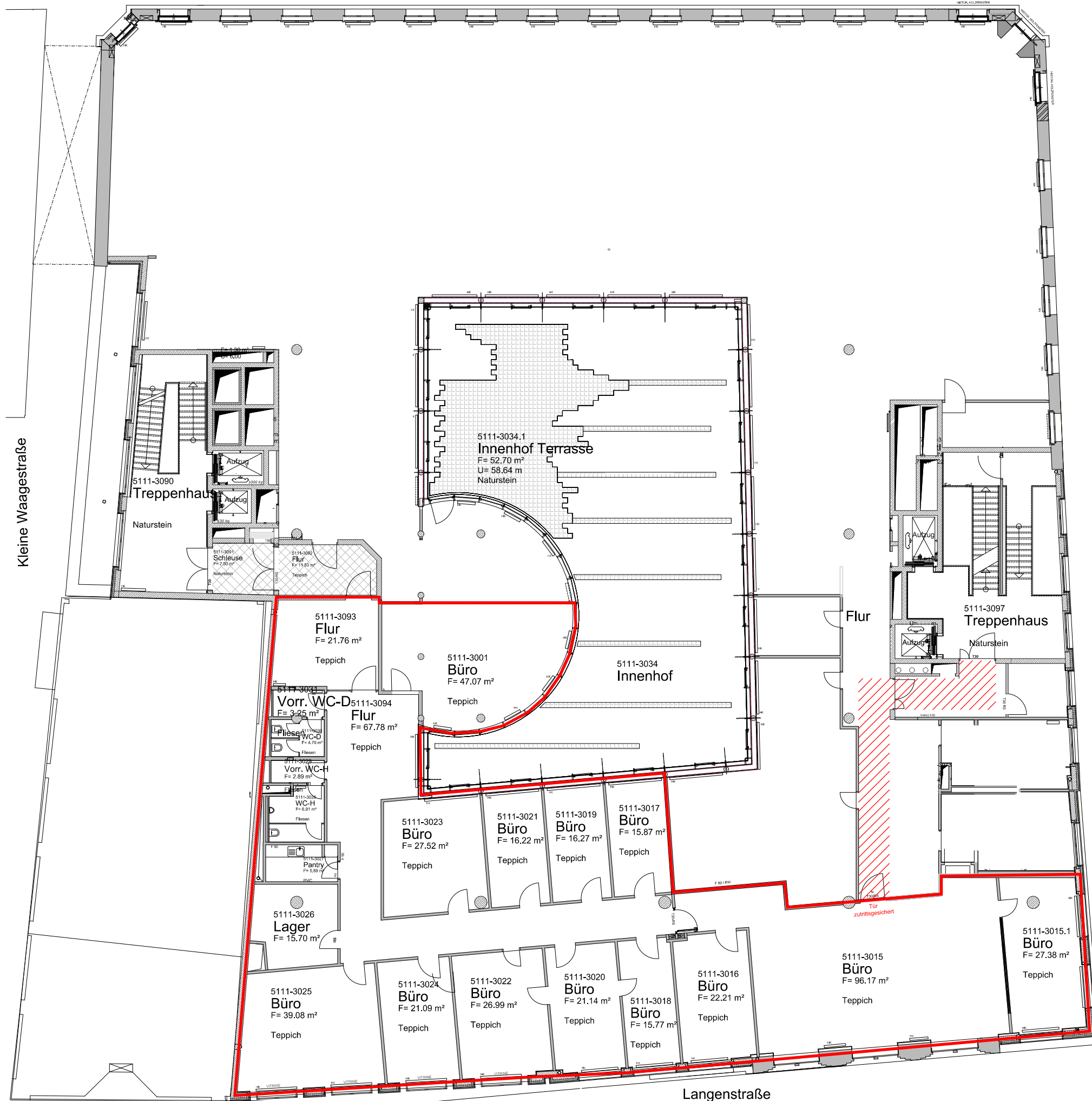
Grundriss 3. Obergeschoss
