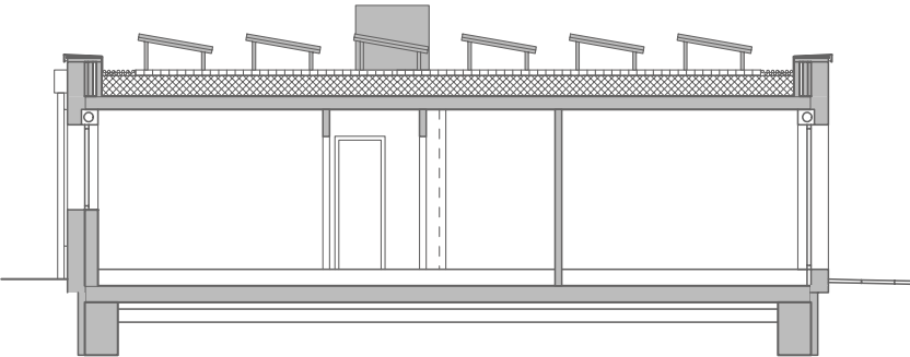
SCHNITT
