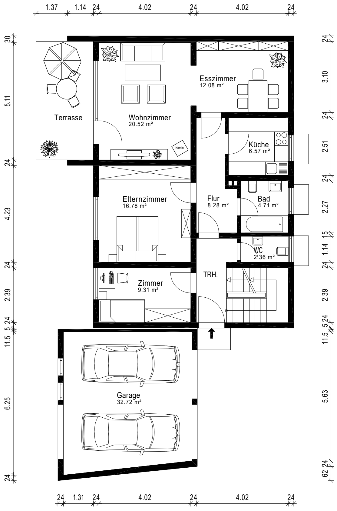
Erdgeschoss
