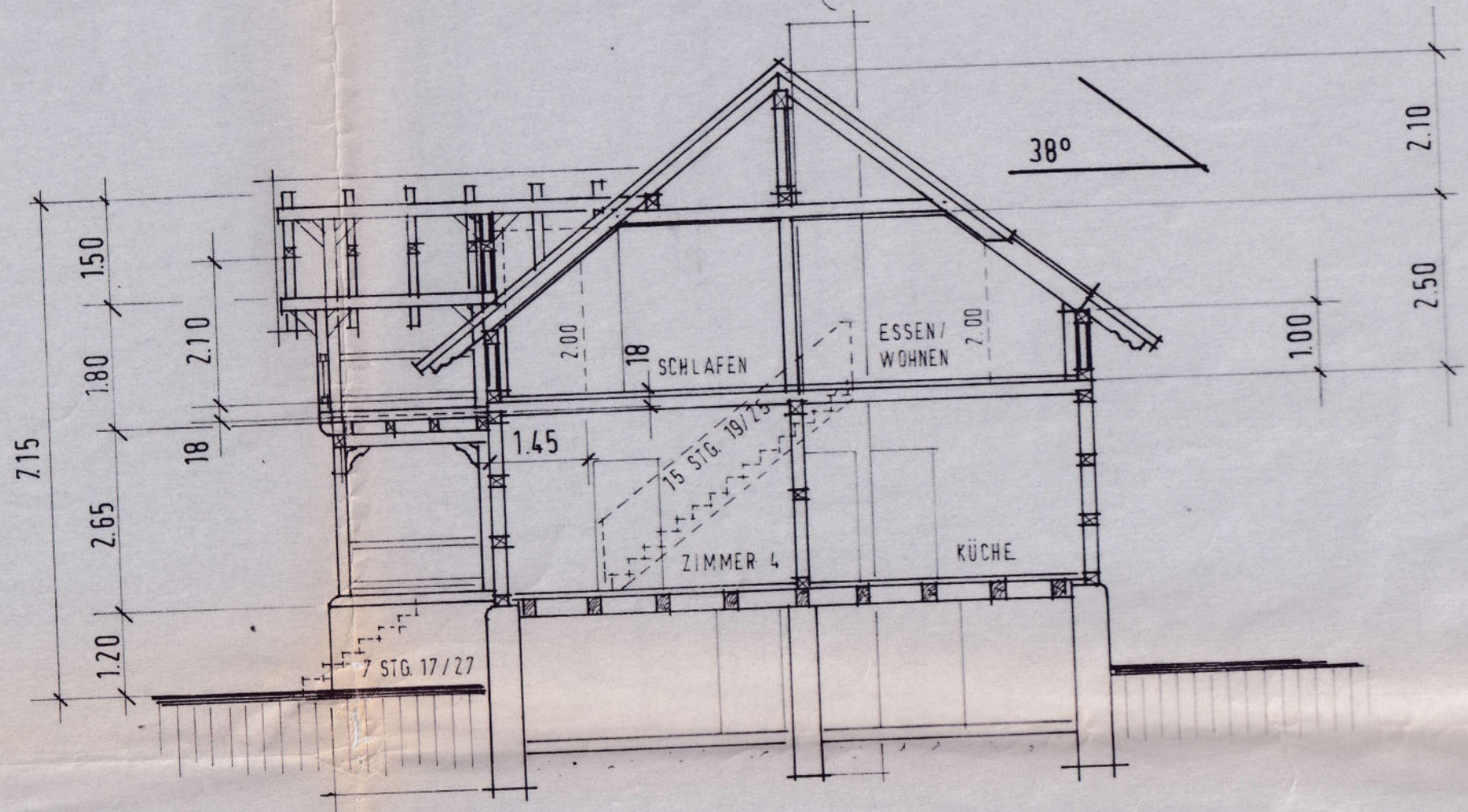
SCHNITT A-A
