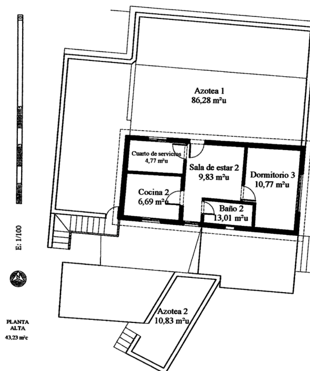
Planta alta vivienda 38011A015003120001WZ (medidas)
