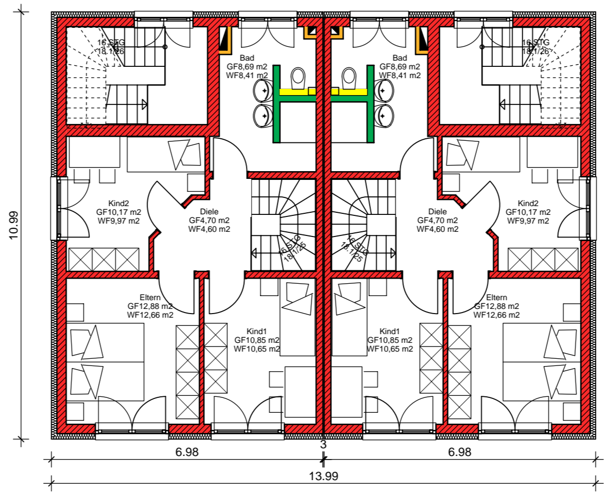
Obergeschoss
