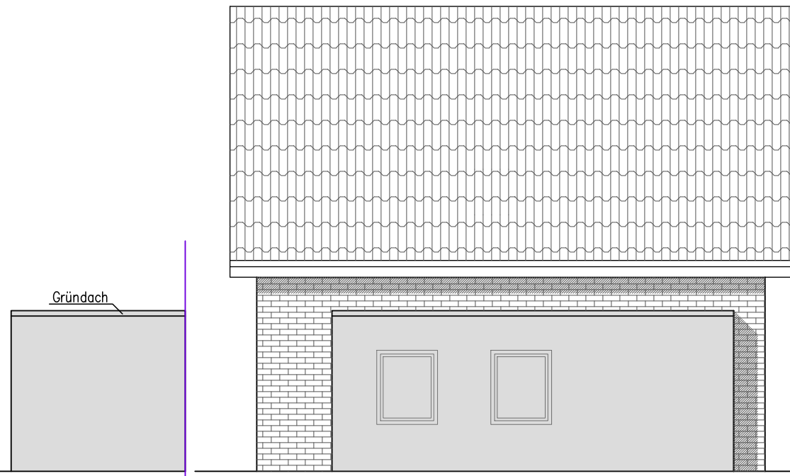
Ansicht Süd-West Grundstück_4
