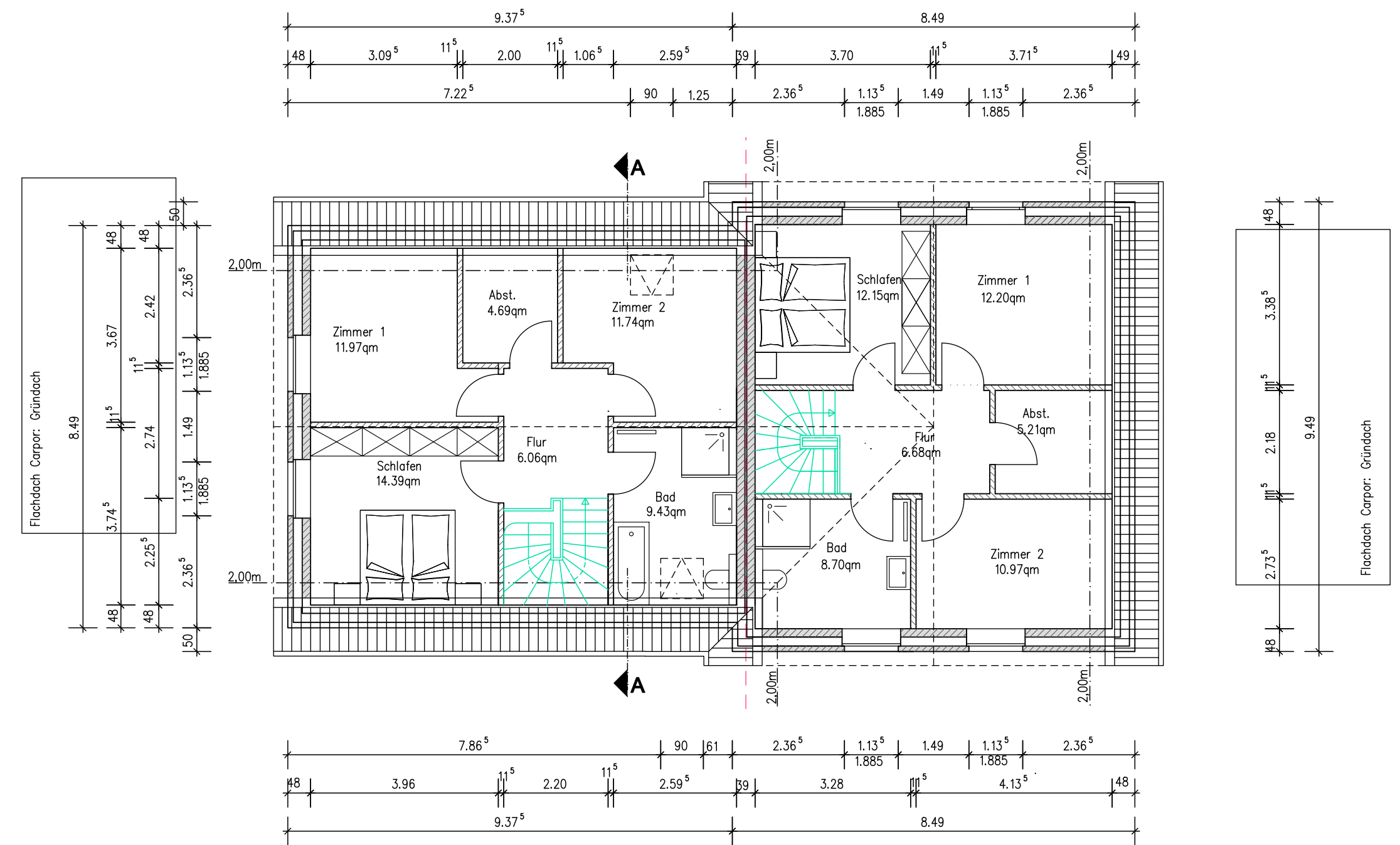
Dachgeschoss Grundstück_4
