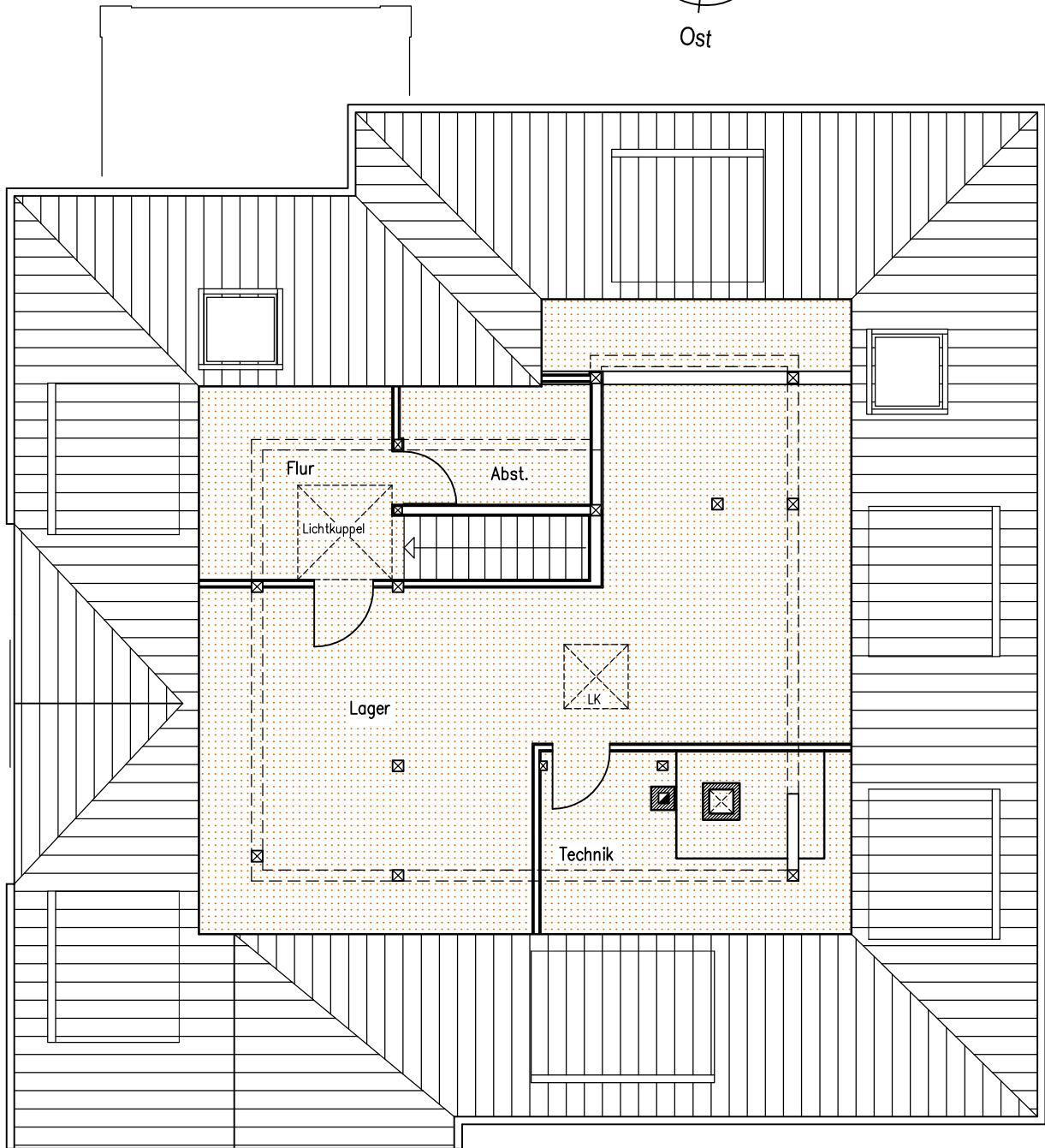
Dachgeschoss
