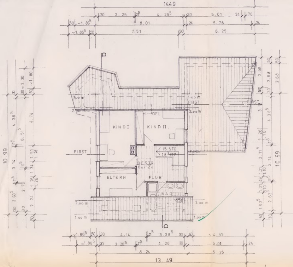
DACHGESCHOSS
