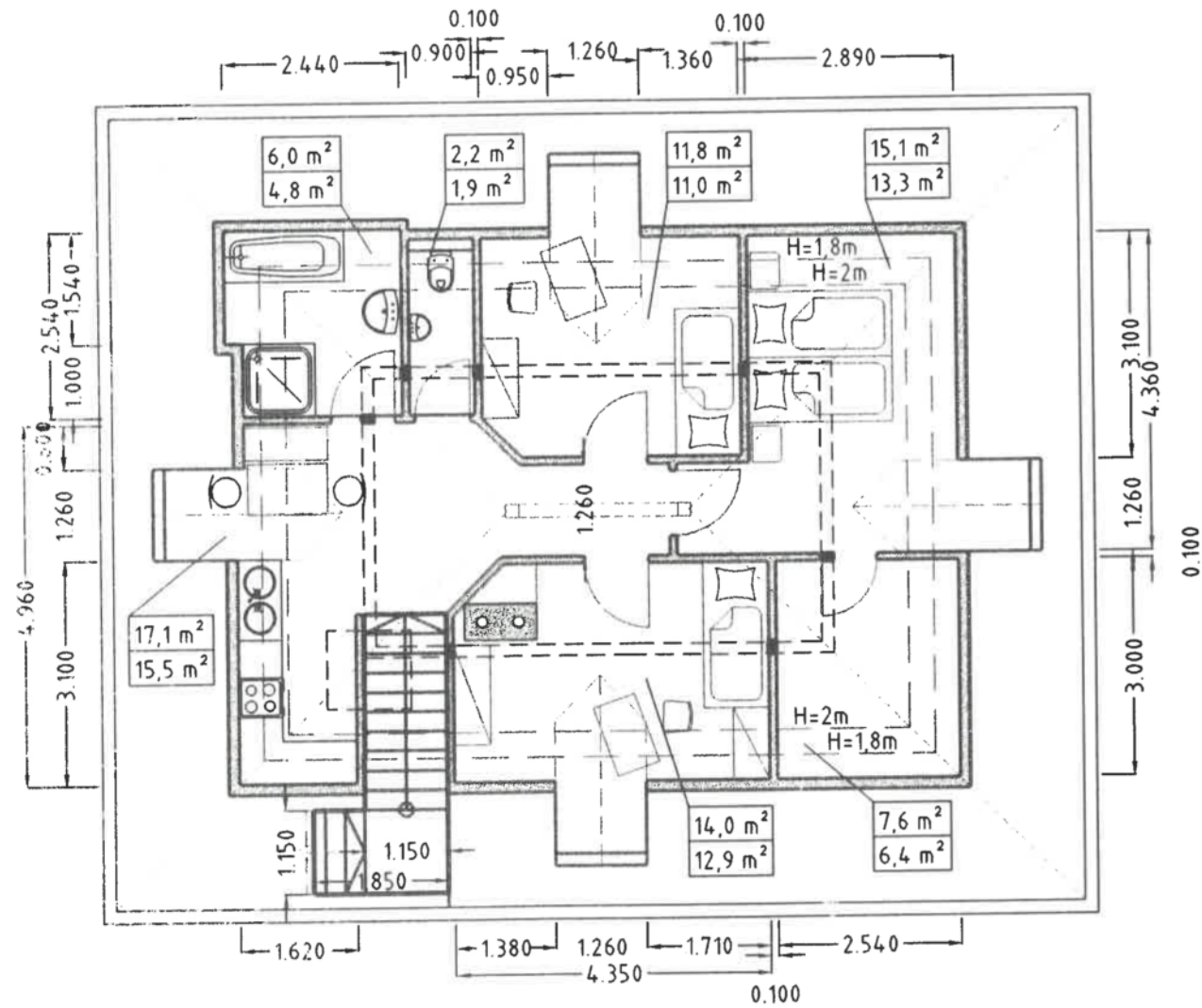
Grundriss Dachgeschoss
