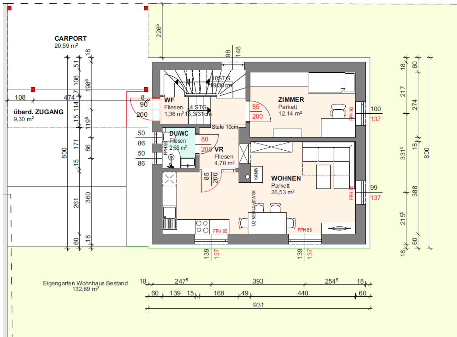
ERDGESCHOSS
