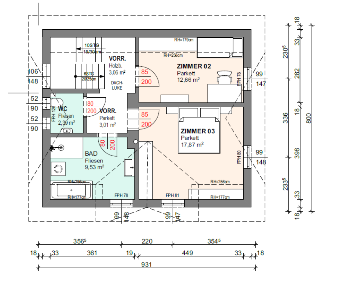
OBERGESCHOSS
