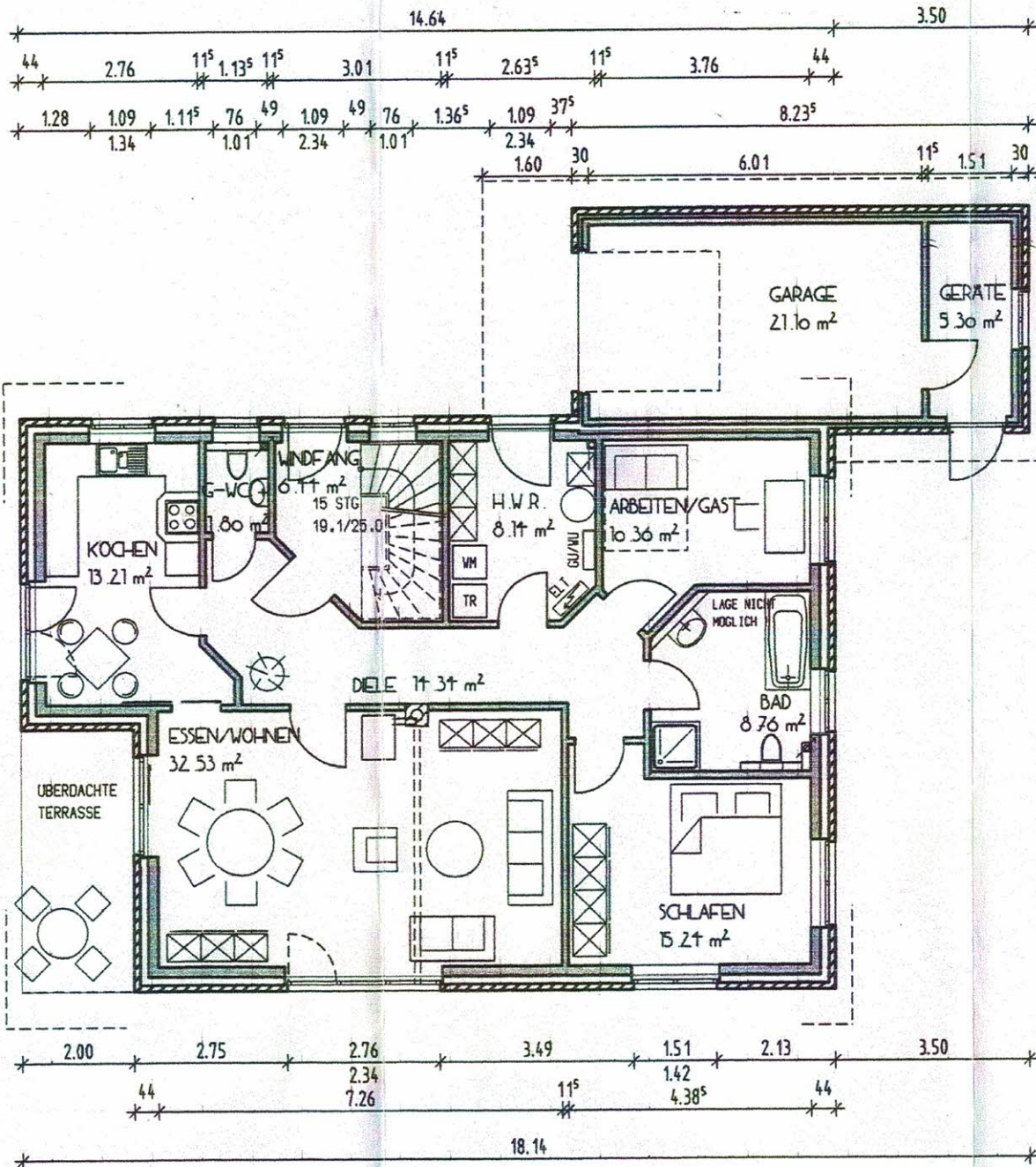
ERDGESCHOSS M 1:100
