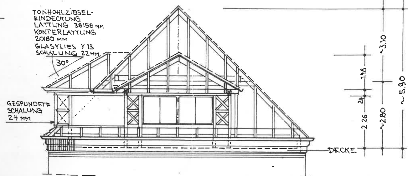
KONSTRUKTIONS-ANSICHT SÜDFASSADE
