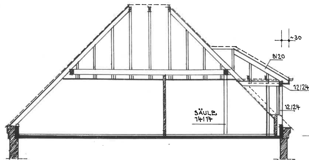
LÄNGSSCHNITT - DACHAUSBAU
