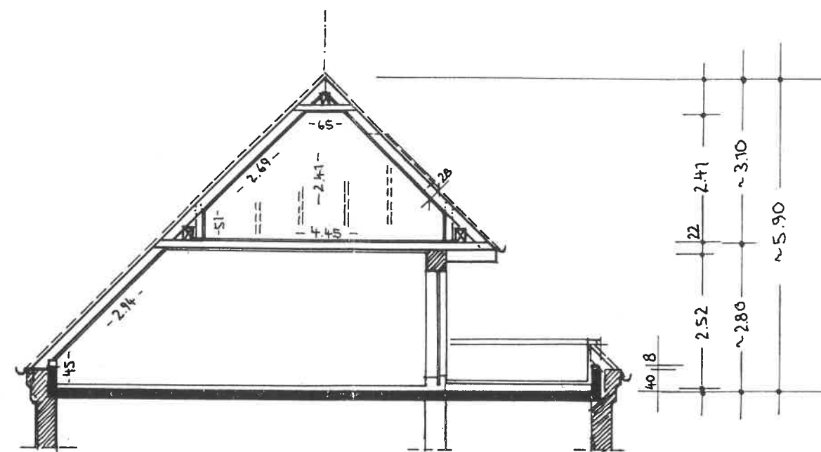
SCHNITT - WOHNRAUM/BALKON (BESTAND)
