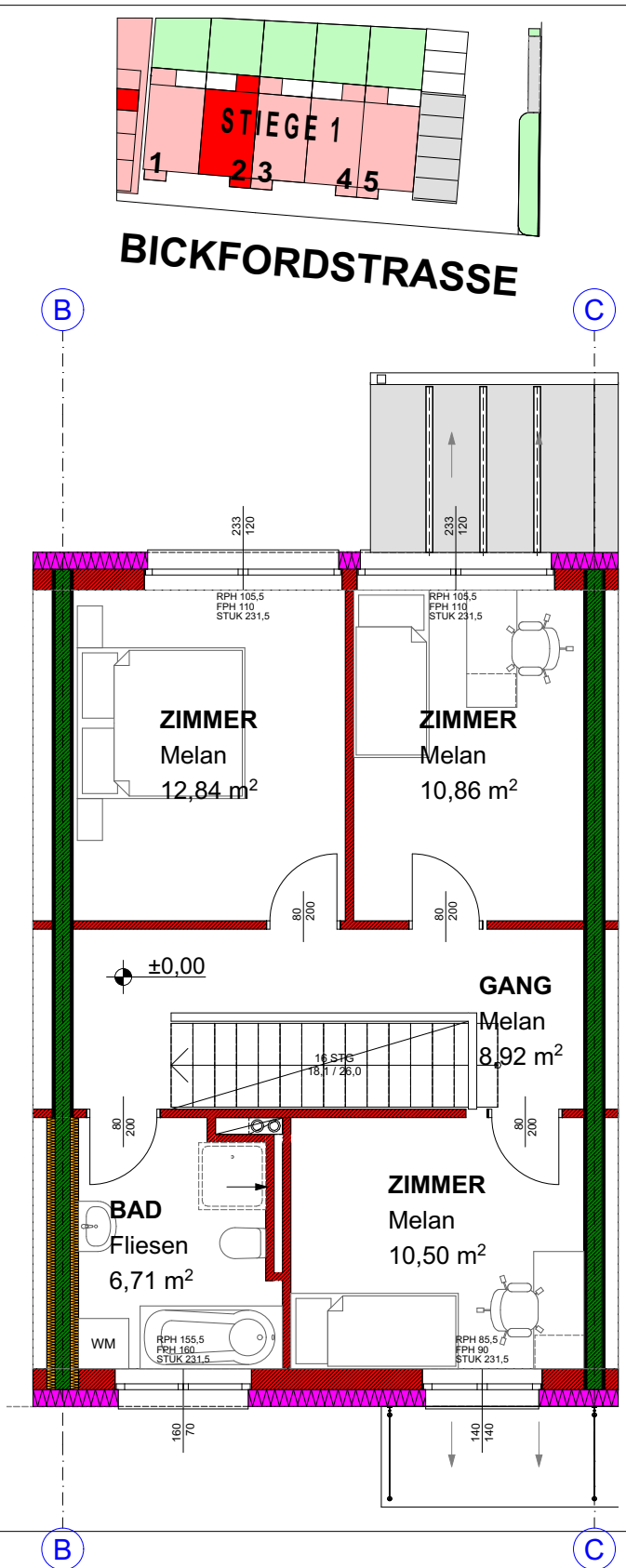
OBERGESCHOSS
