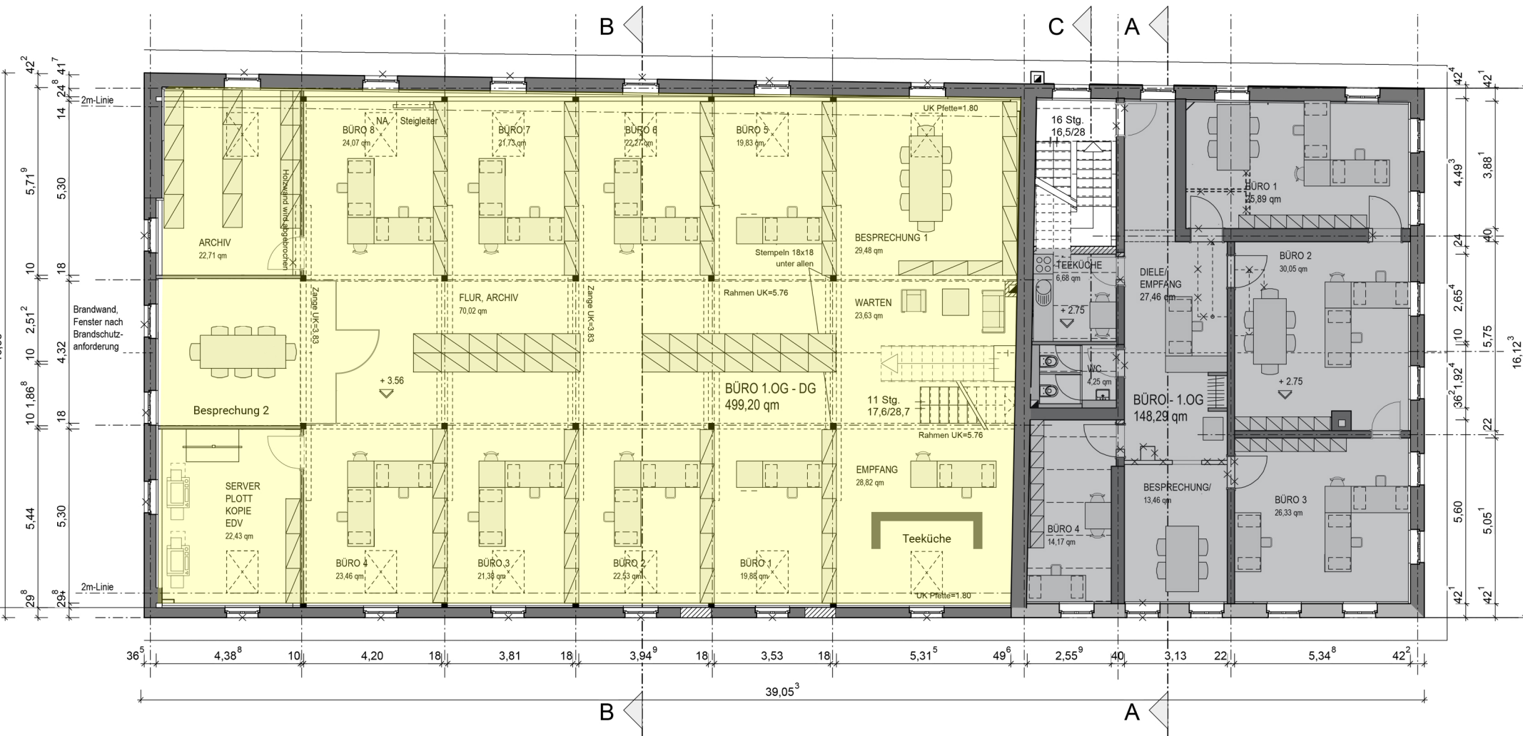
GRUNDRISS 1.OBERGESCHOSS
