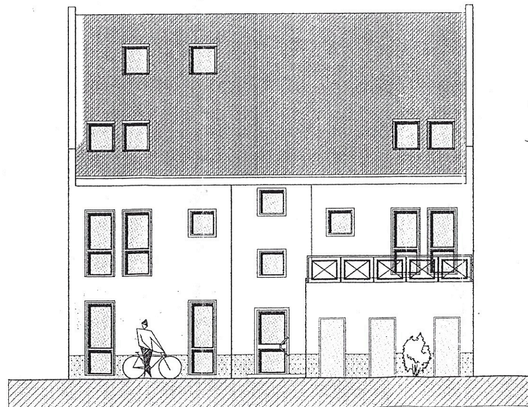
ANSICHT SÜD-WEST (HOFSEITE)
