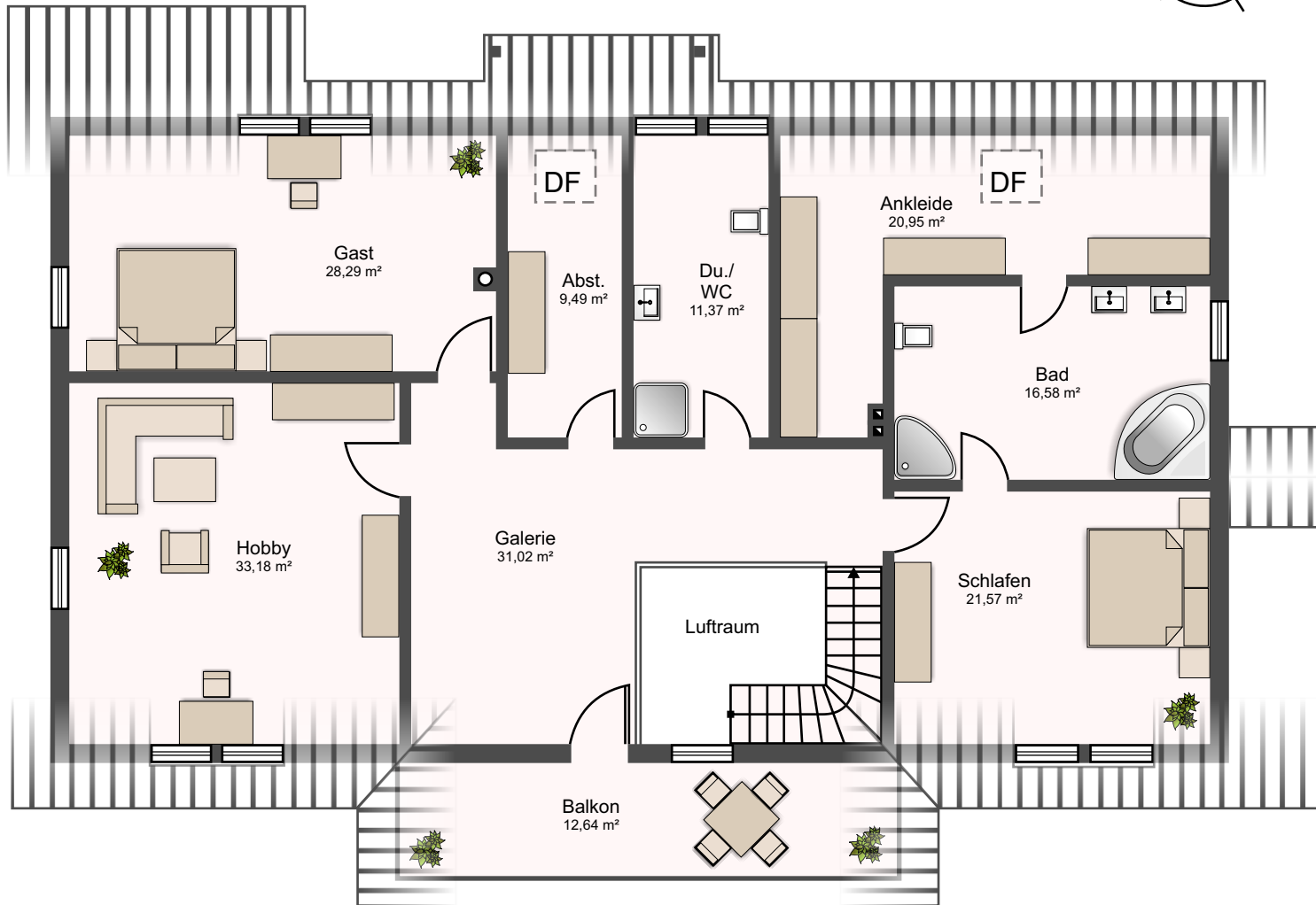
Dachgeschoss
