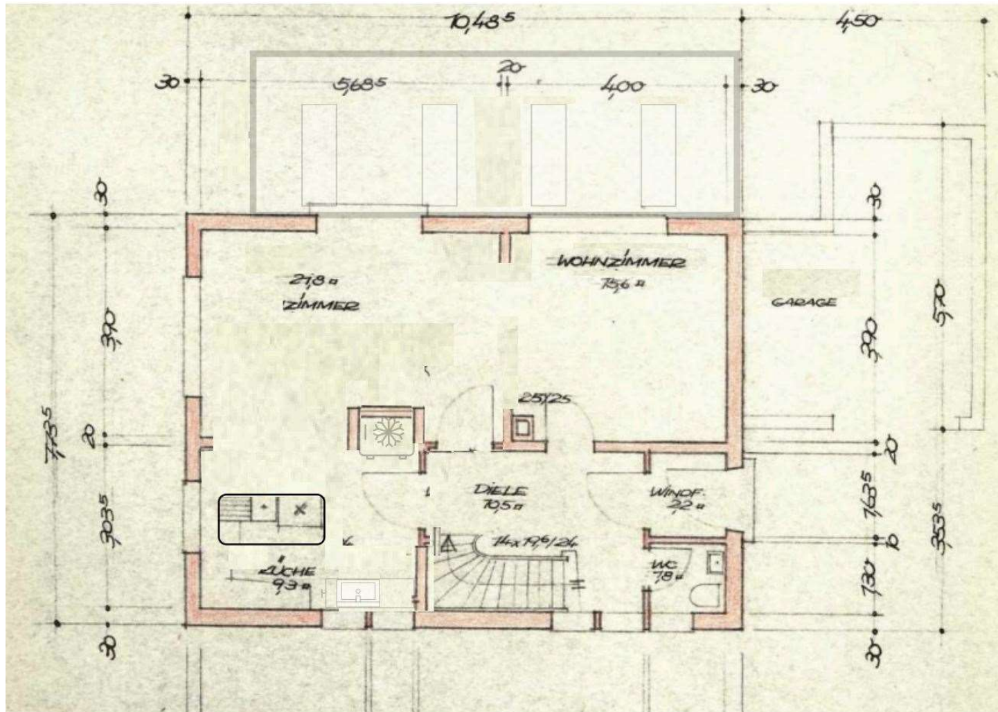
Grundriss EG
