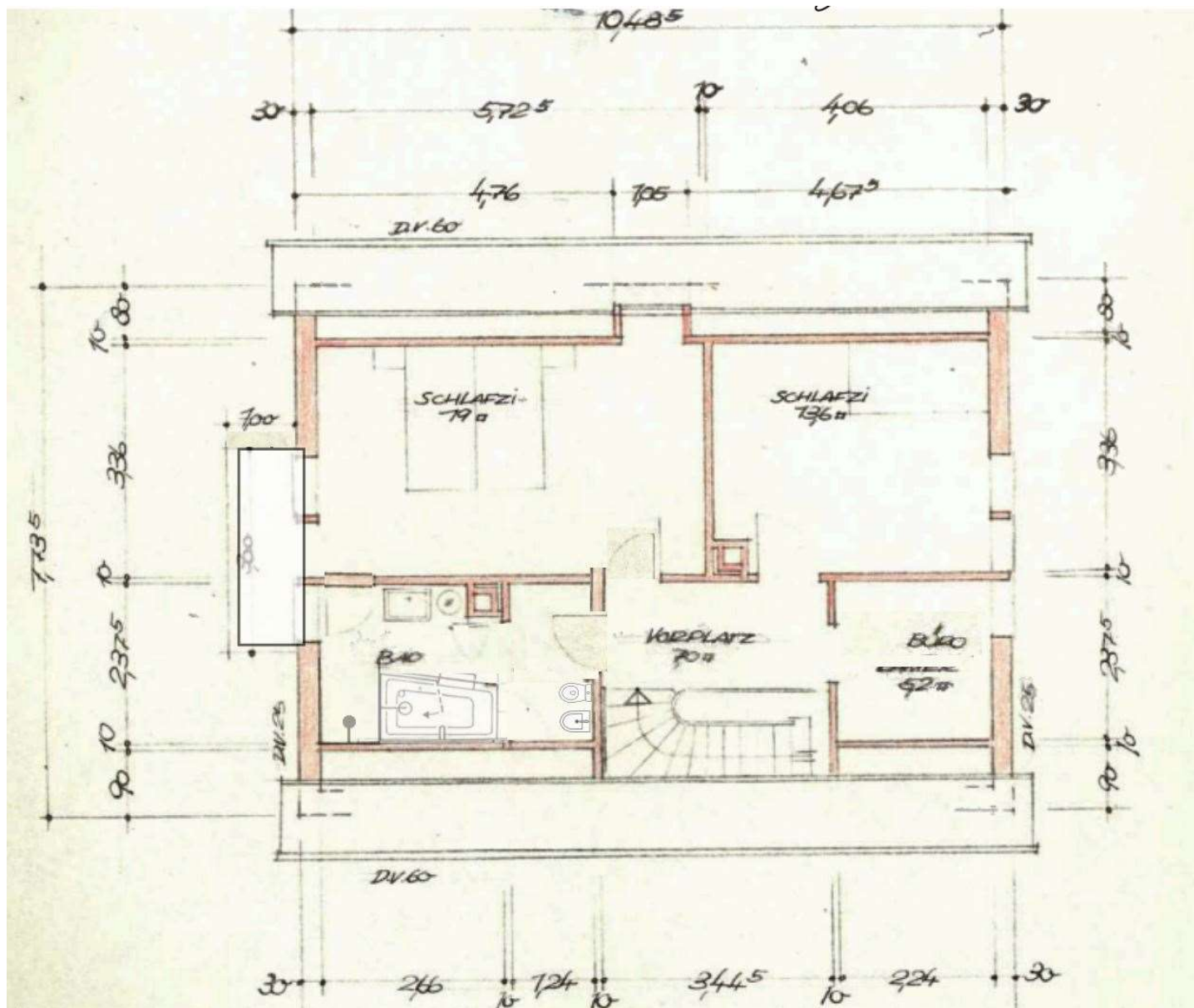
Grundriss OG
