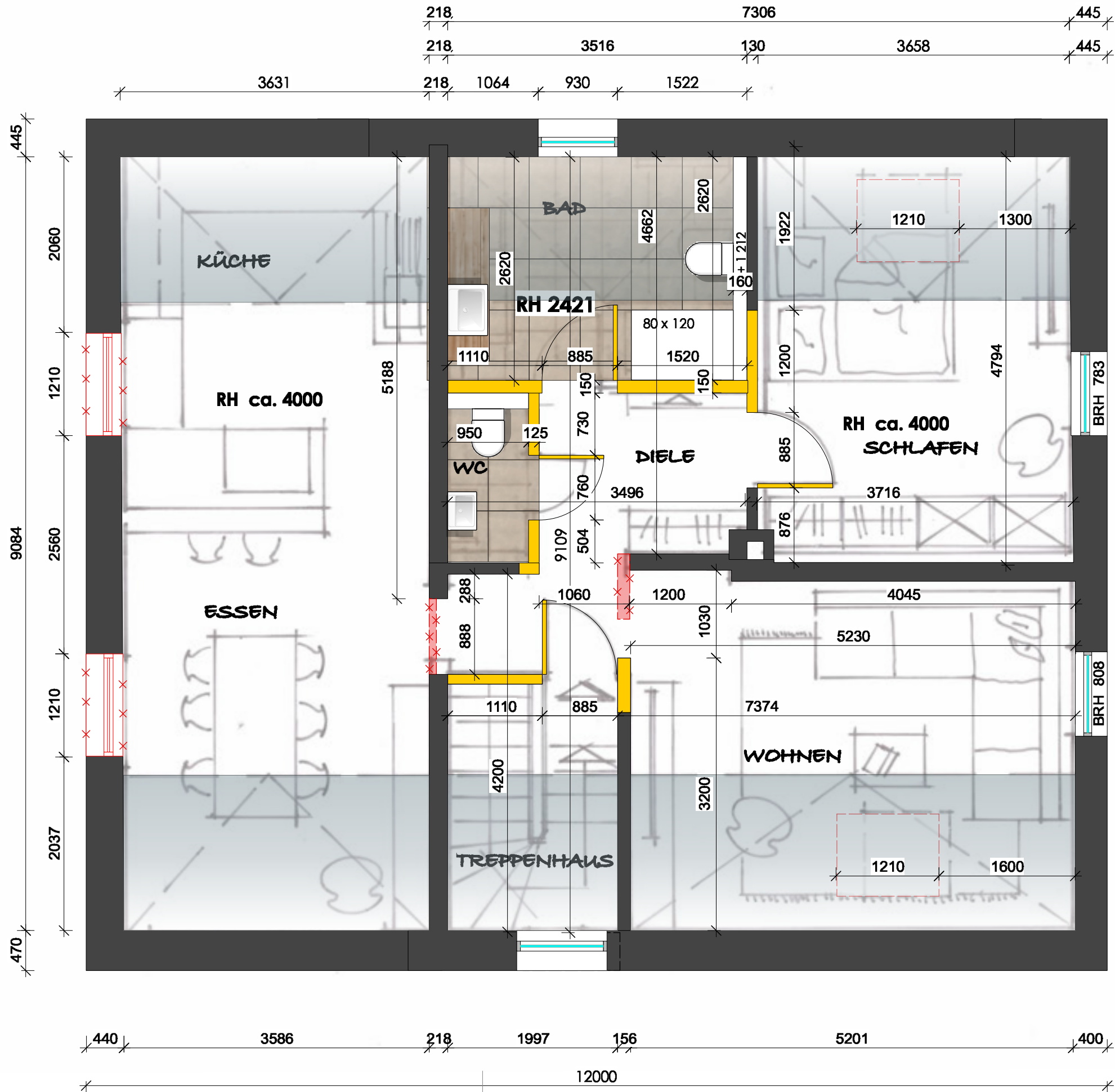
OBERGESCHOSS GRUNDRISS - Wohnung B
