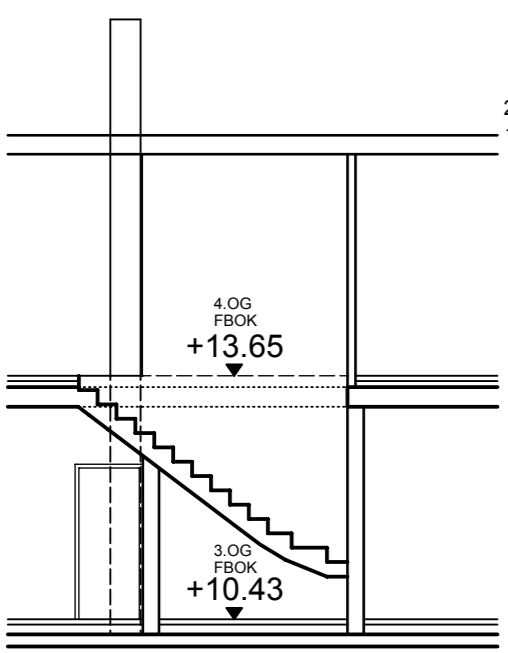
HILFSSCHNITT DURCH STIEGE WE 2
