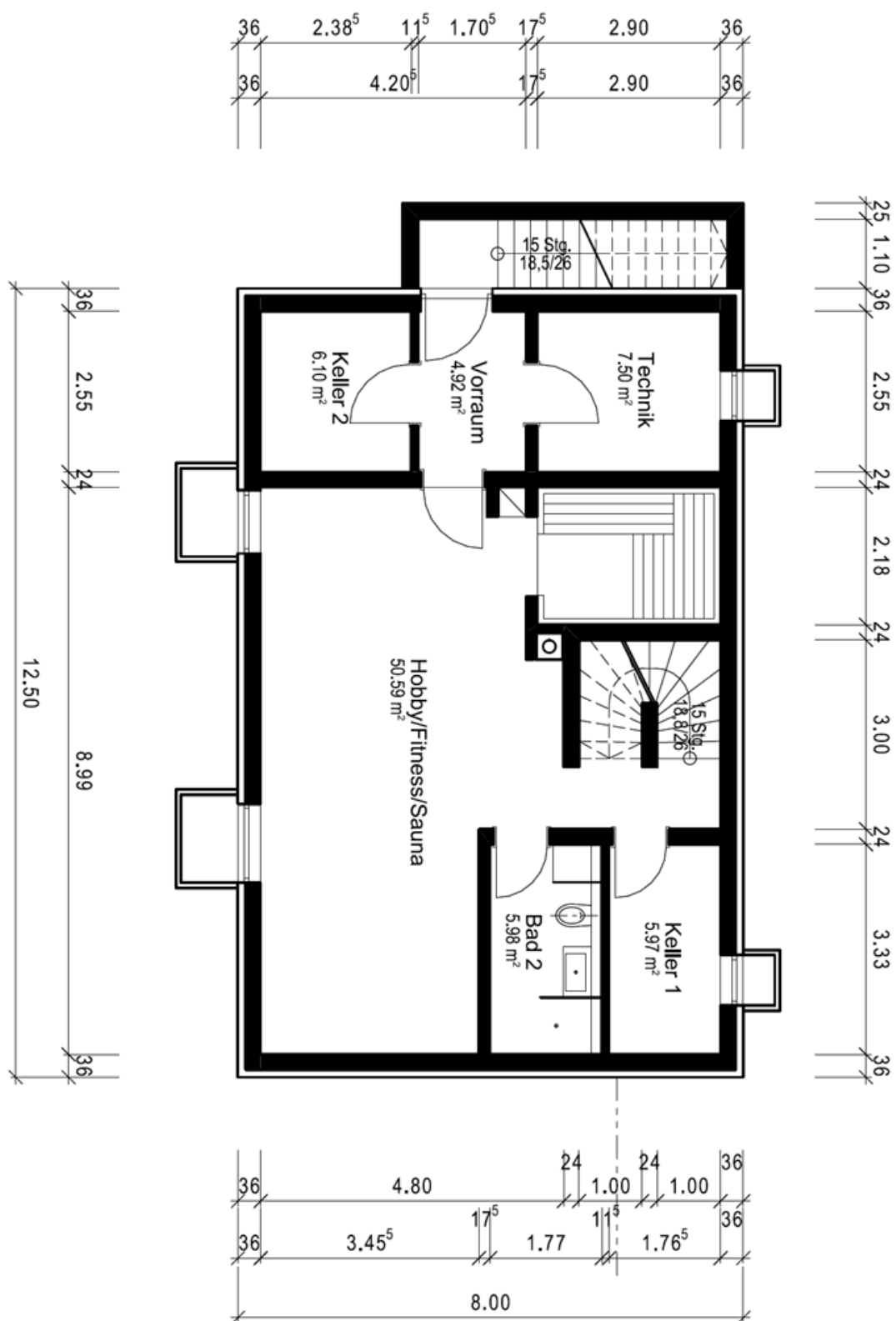
Grundriss UG
