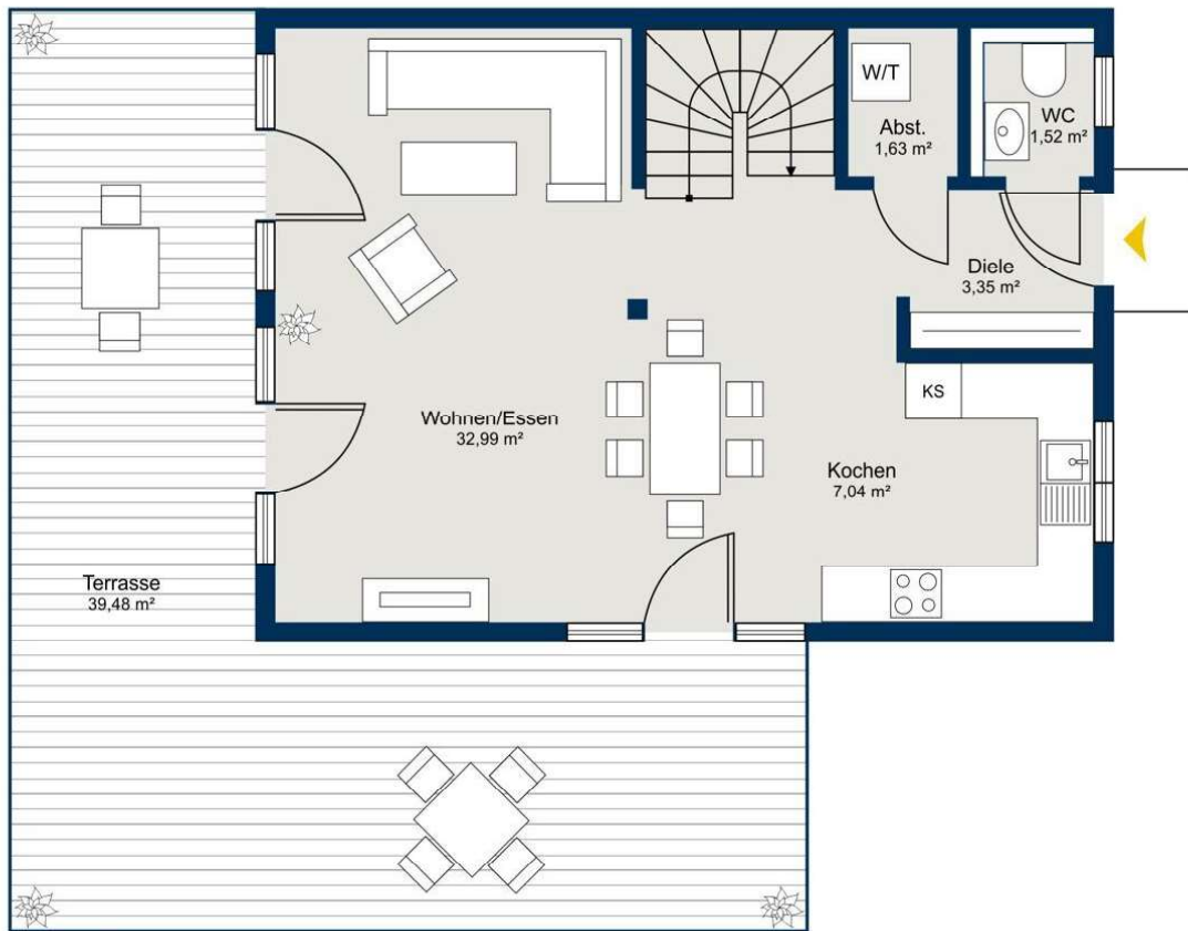
Grundriss Erdgeschoss
