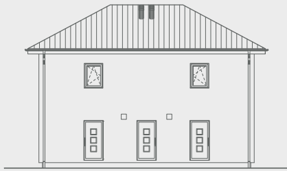
Ansicht Eingang
