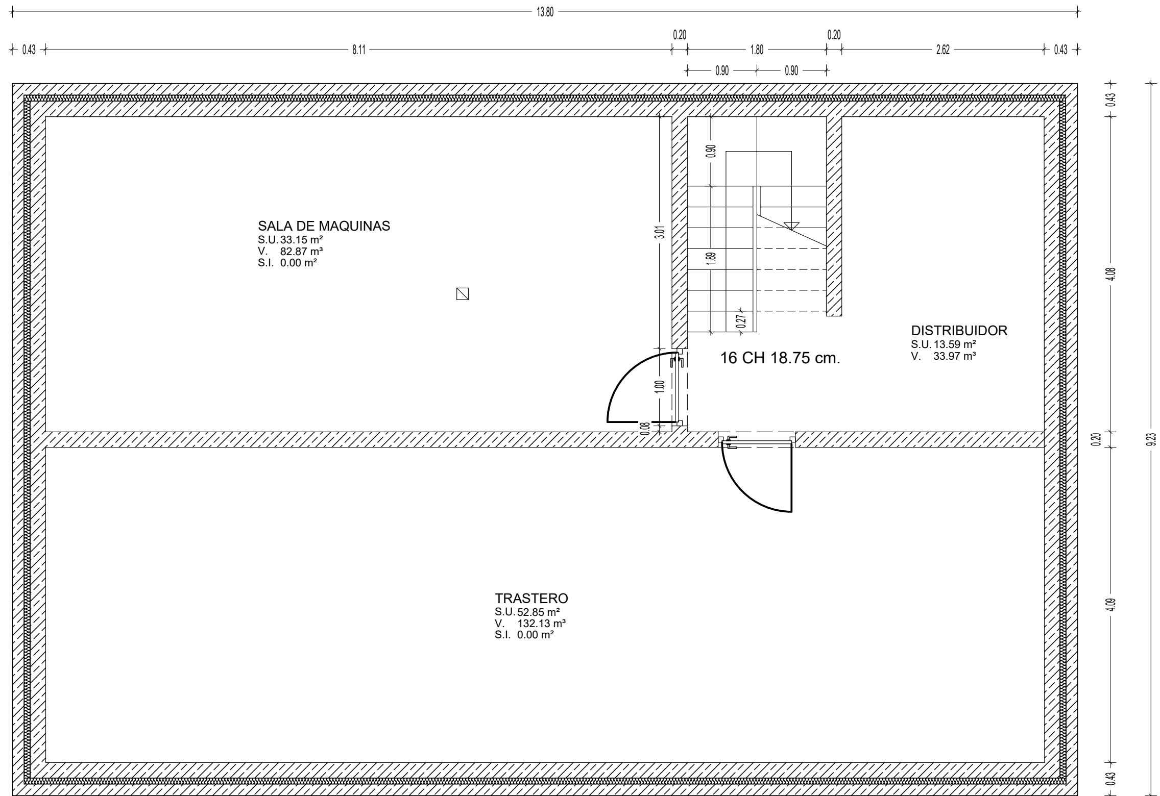
PL. SOTANO
