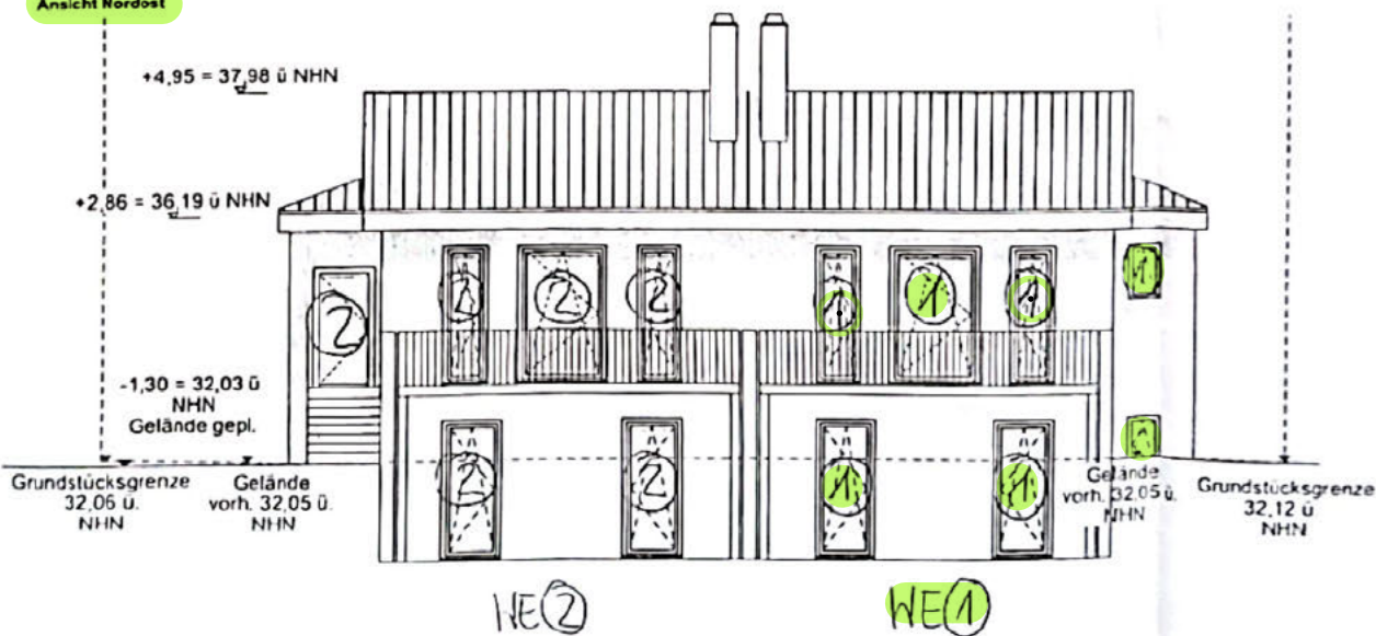
Ansicht Nordost
