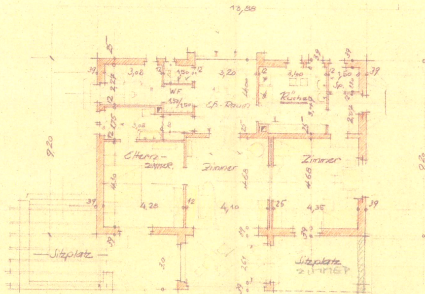
Erdgeschoss
