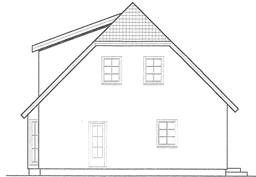
Ansicht Süd
