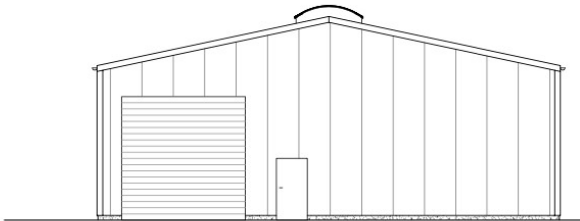
Nordostansicht (Achse 7)
