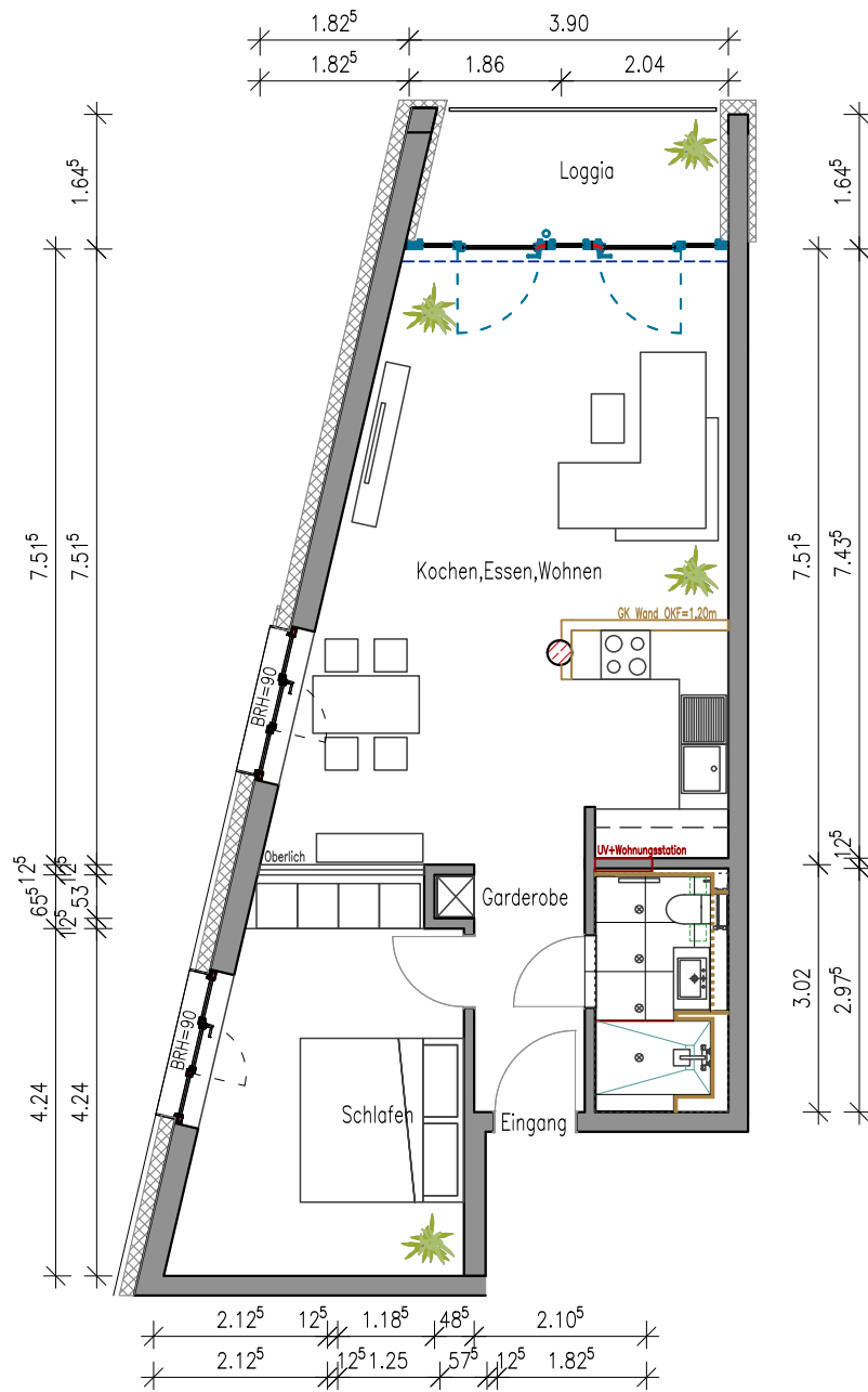
WOHNUNGSTYP III M1:100
