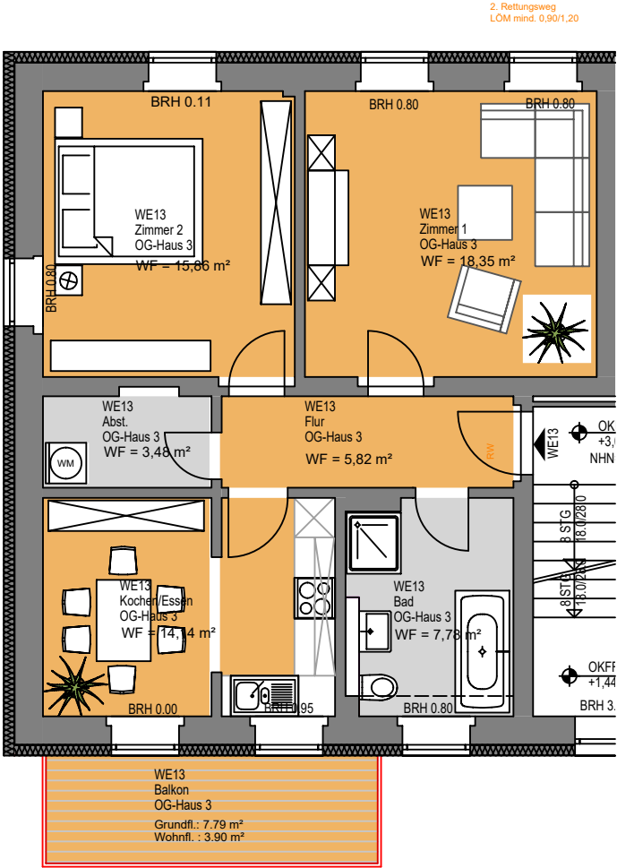
Obergeschoss WE13
