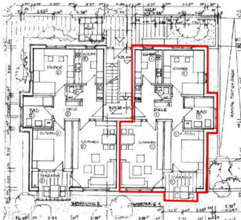
Grundriss Erdgeschoss, ETW Nr. 1 rot umrandet
