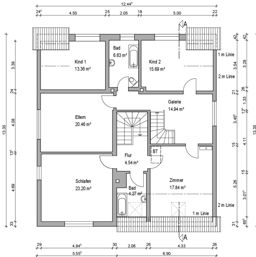
Grundriss Obergeschoss
