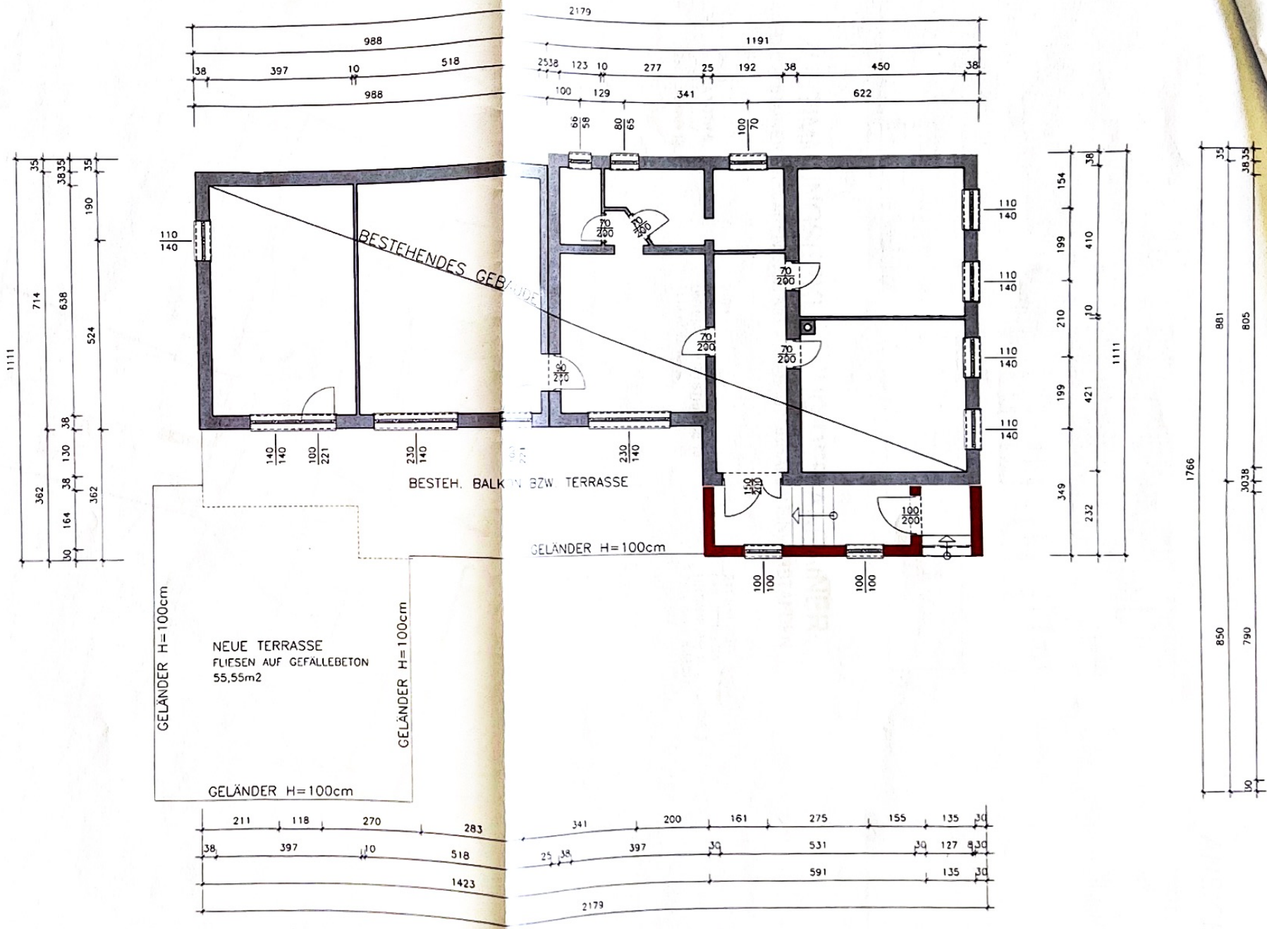
GRUNDRISS ERDGESCHOSS
