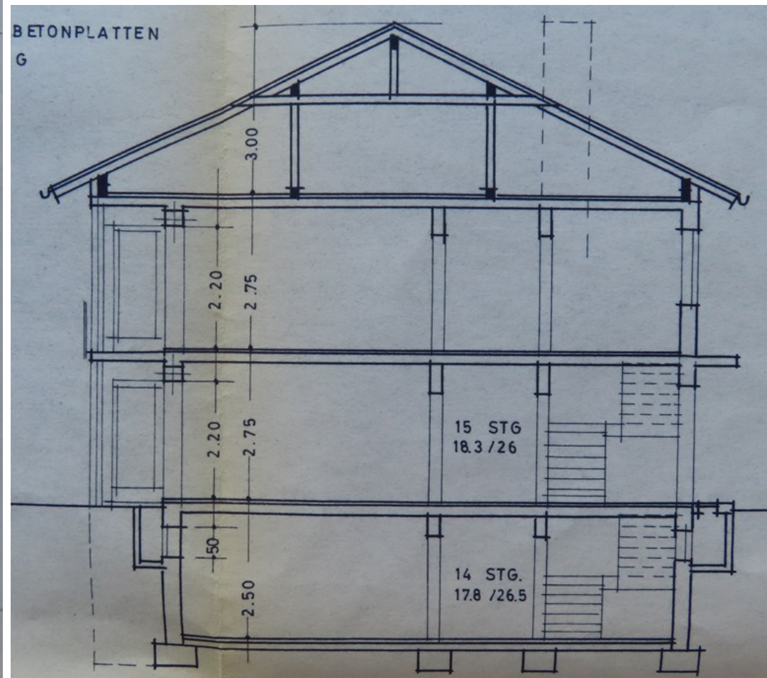
Schnitt vom Haus
