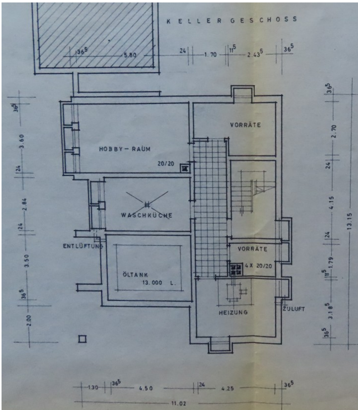
Plan vom Keller
