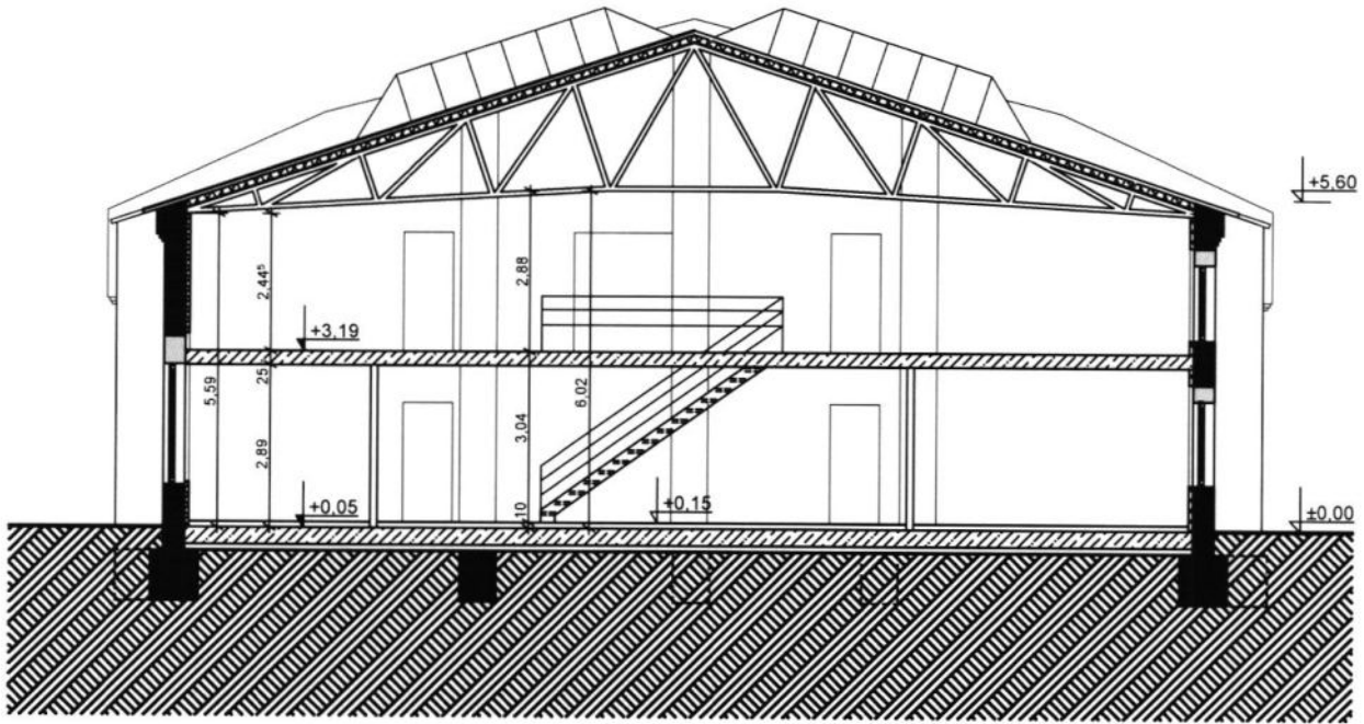
Schnitt B-B
