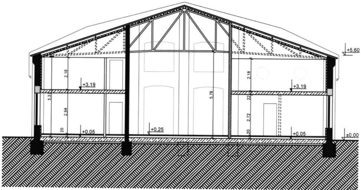
Schnitt A-A
