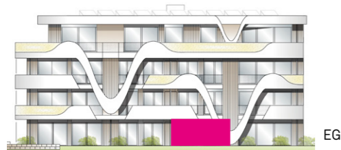
Haus E - Ansicht Süd
