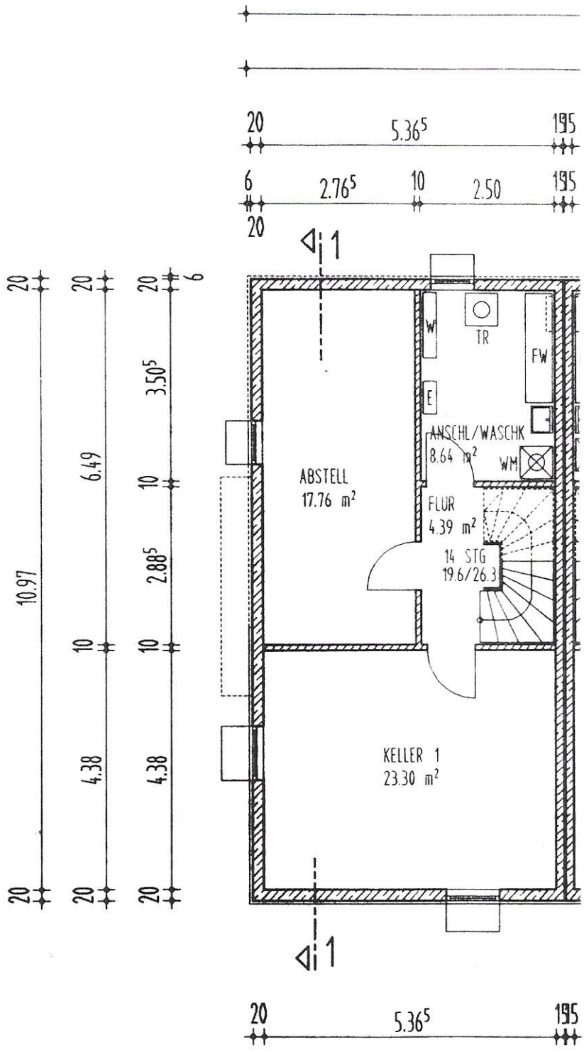
KELLERGESCHOSS HAUS 15 TYP "A1"
