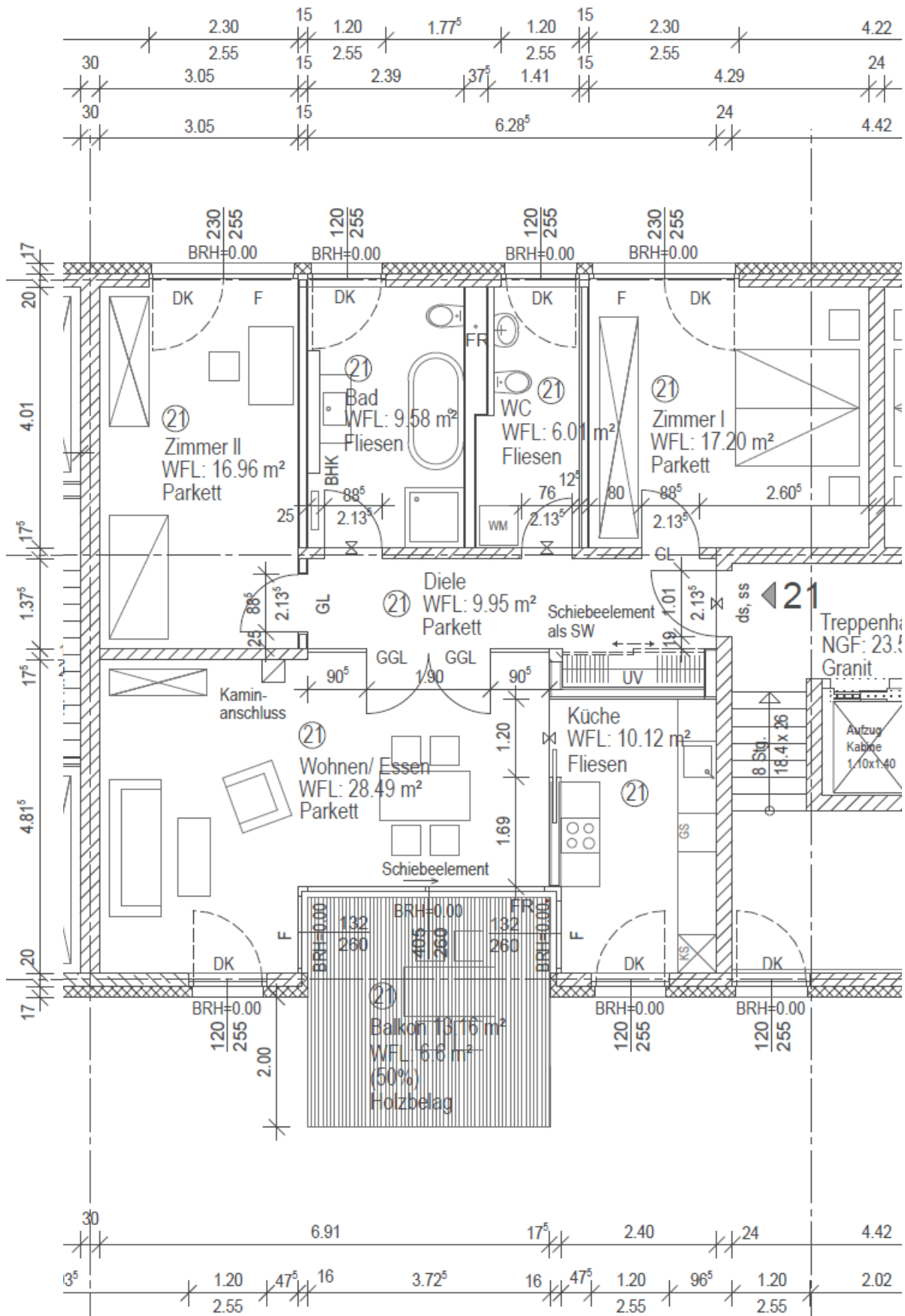
Grundriss Wohnung 21
