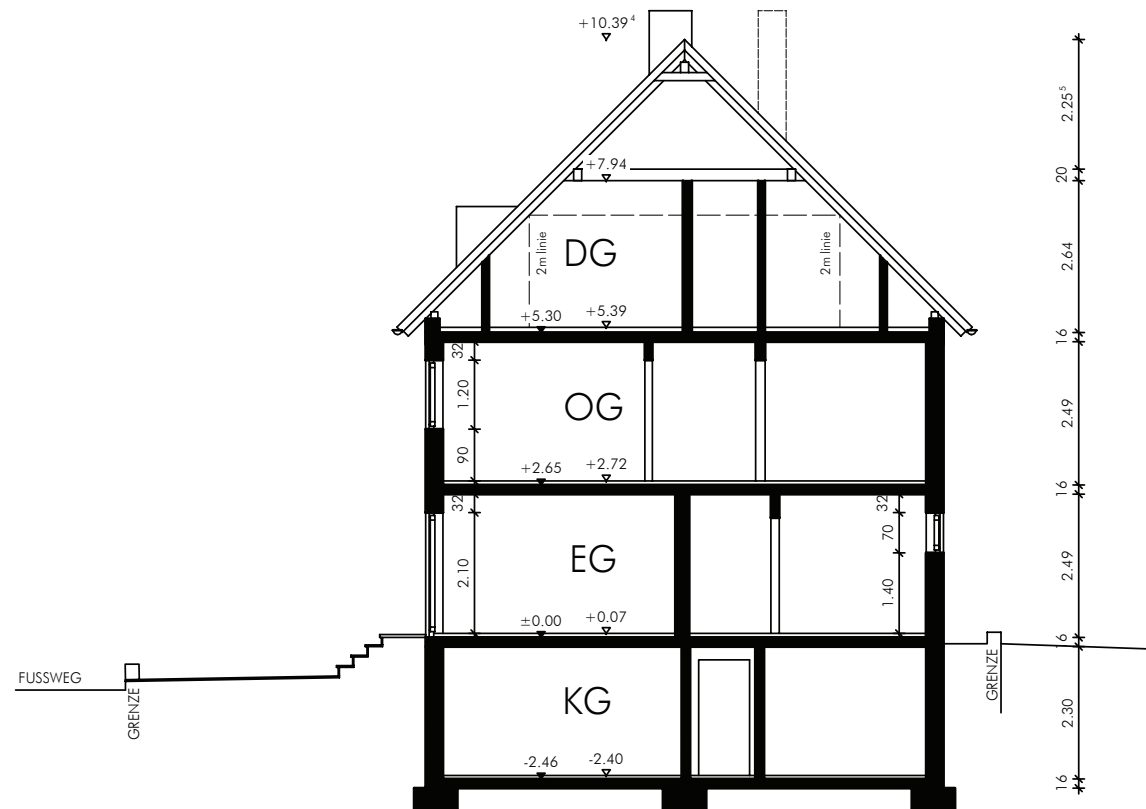
SCHNITT A-A
