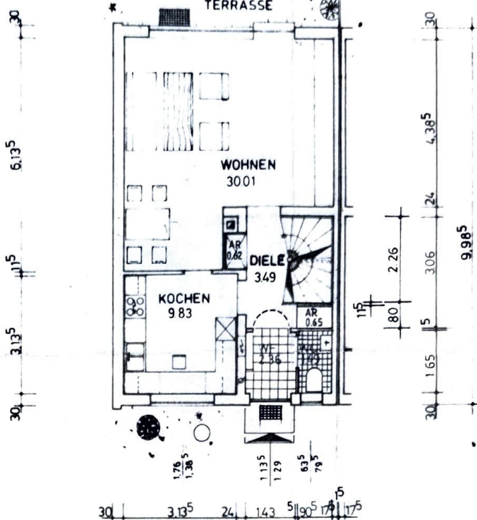
ERDGESCHOSS
