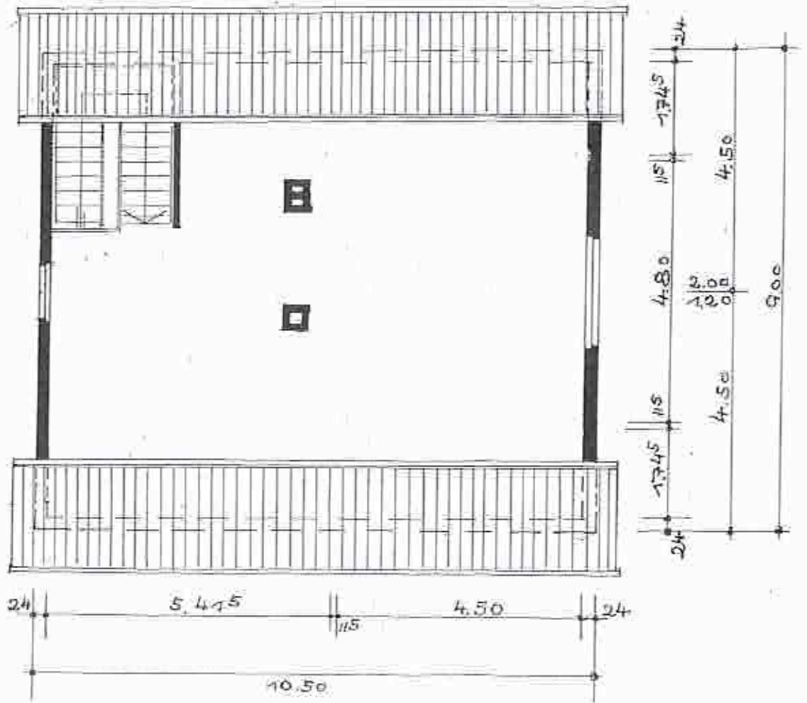
DACHGESCHOSS
