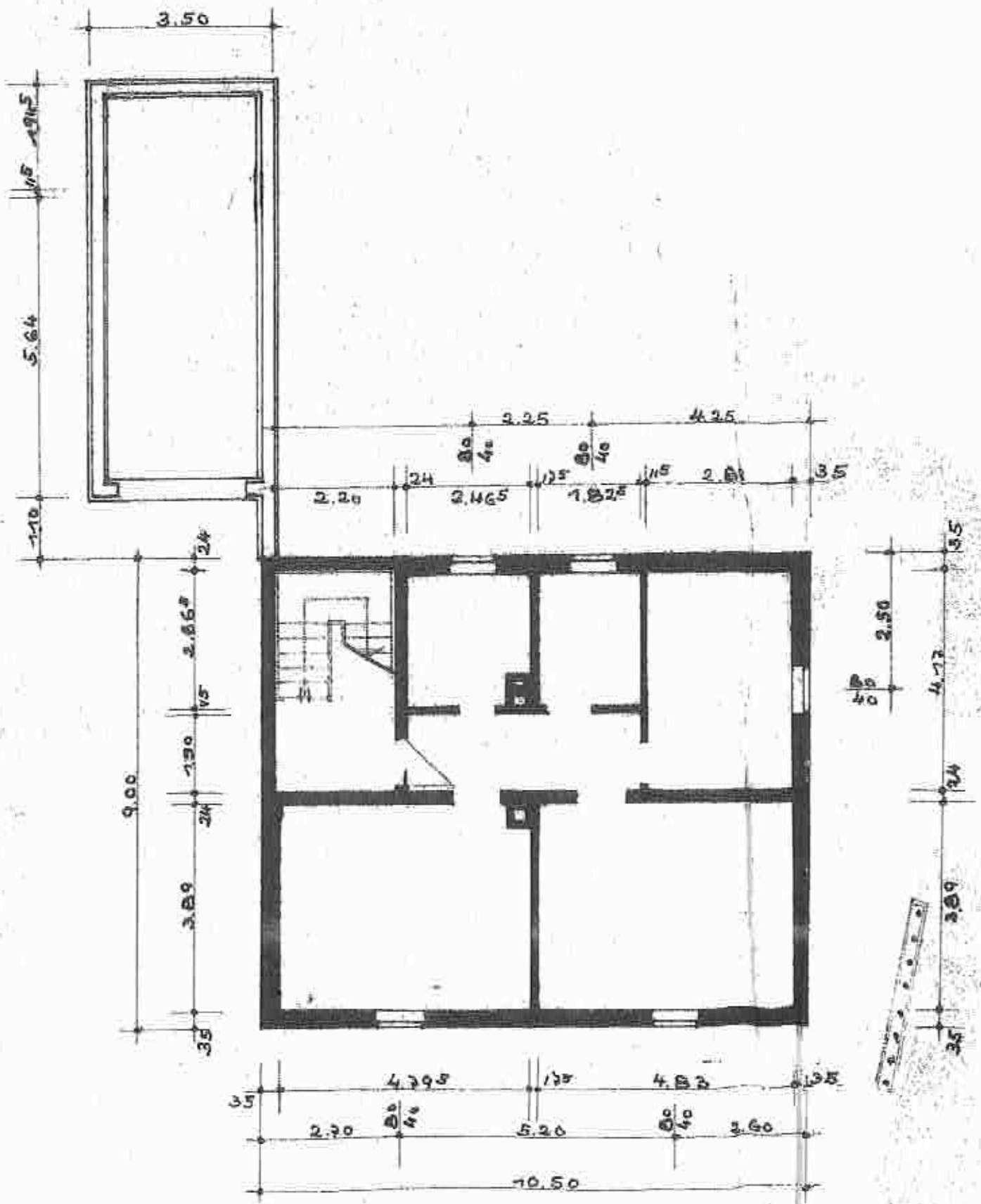
KELLERGESCHOSS
