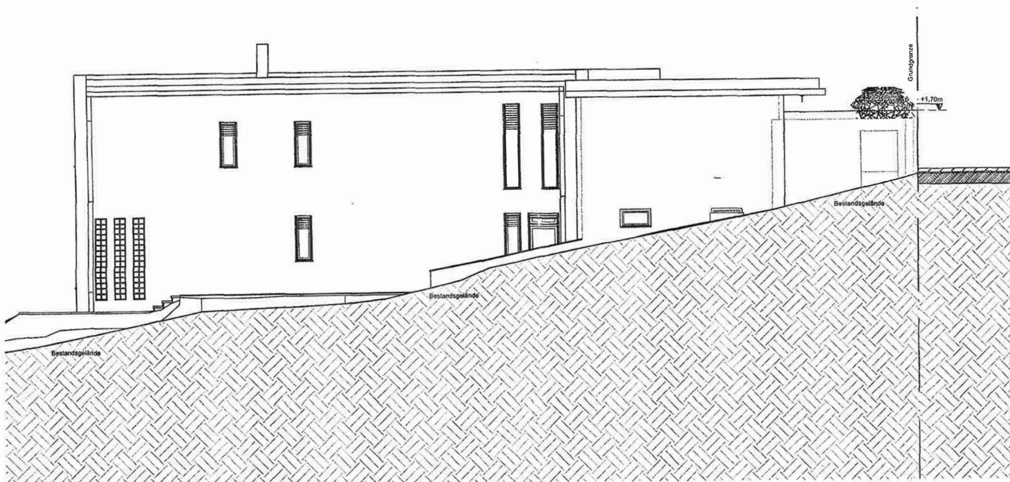
ANSICHT NORD
