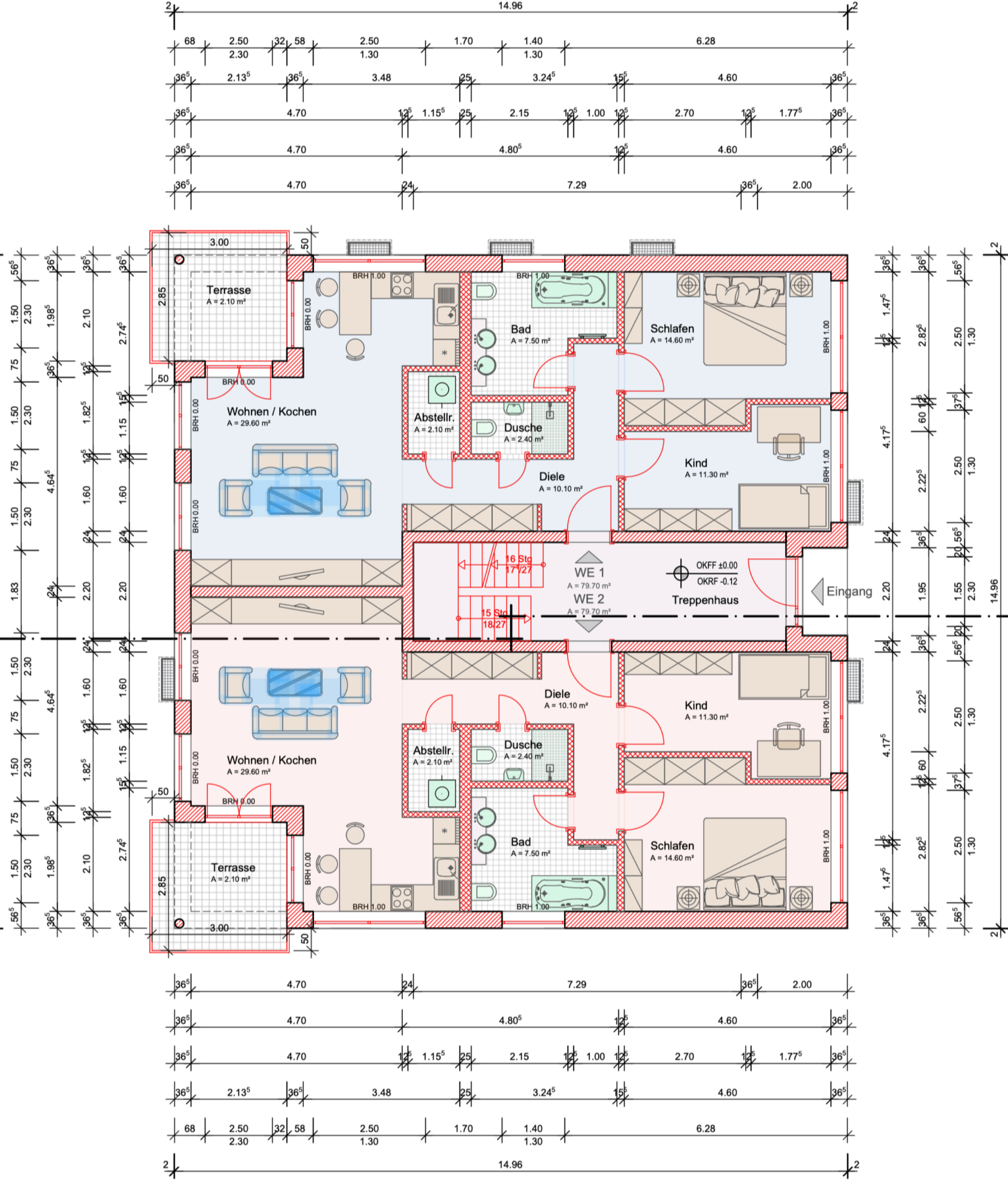
Grundriss Erdgeschoss
