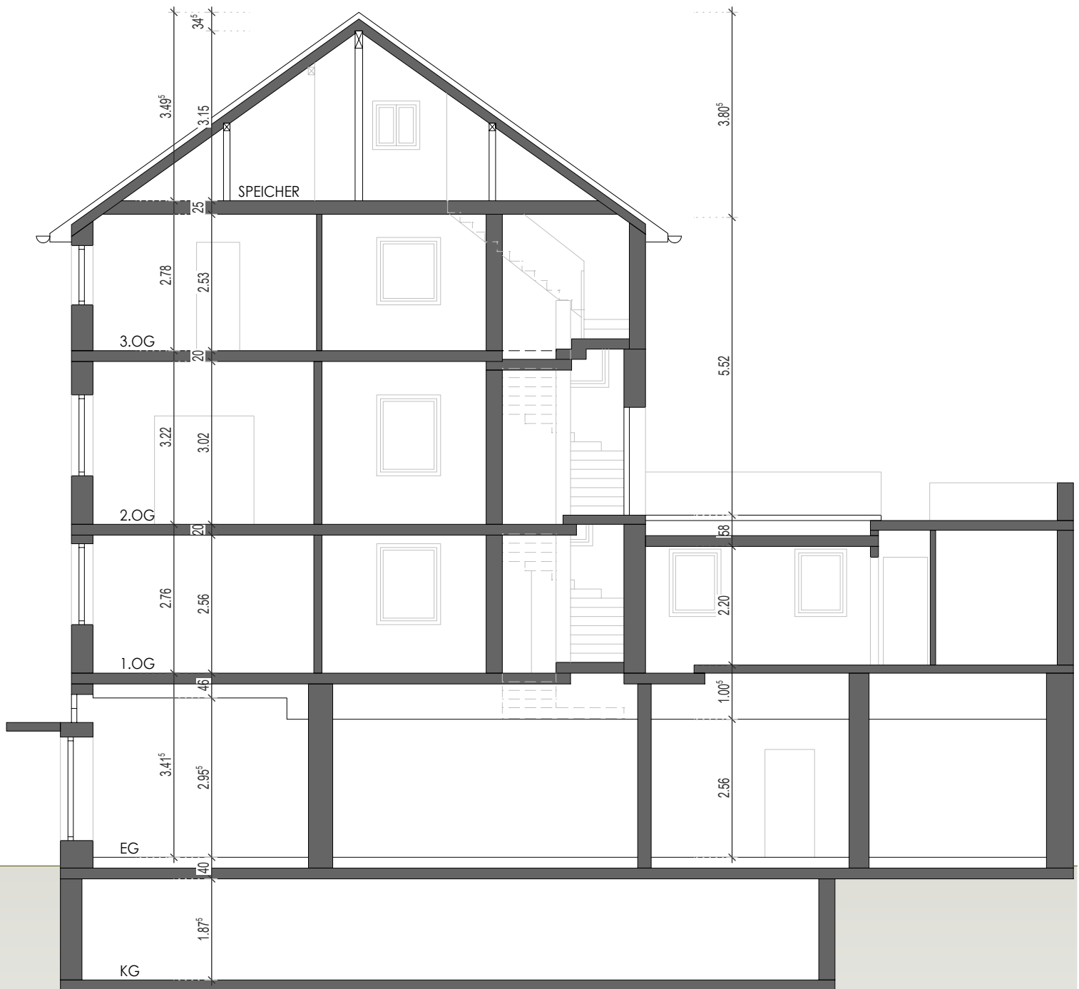
QUERSCHNITT
