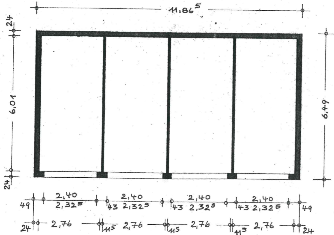
GRUNDRISS
