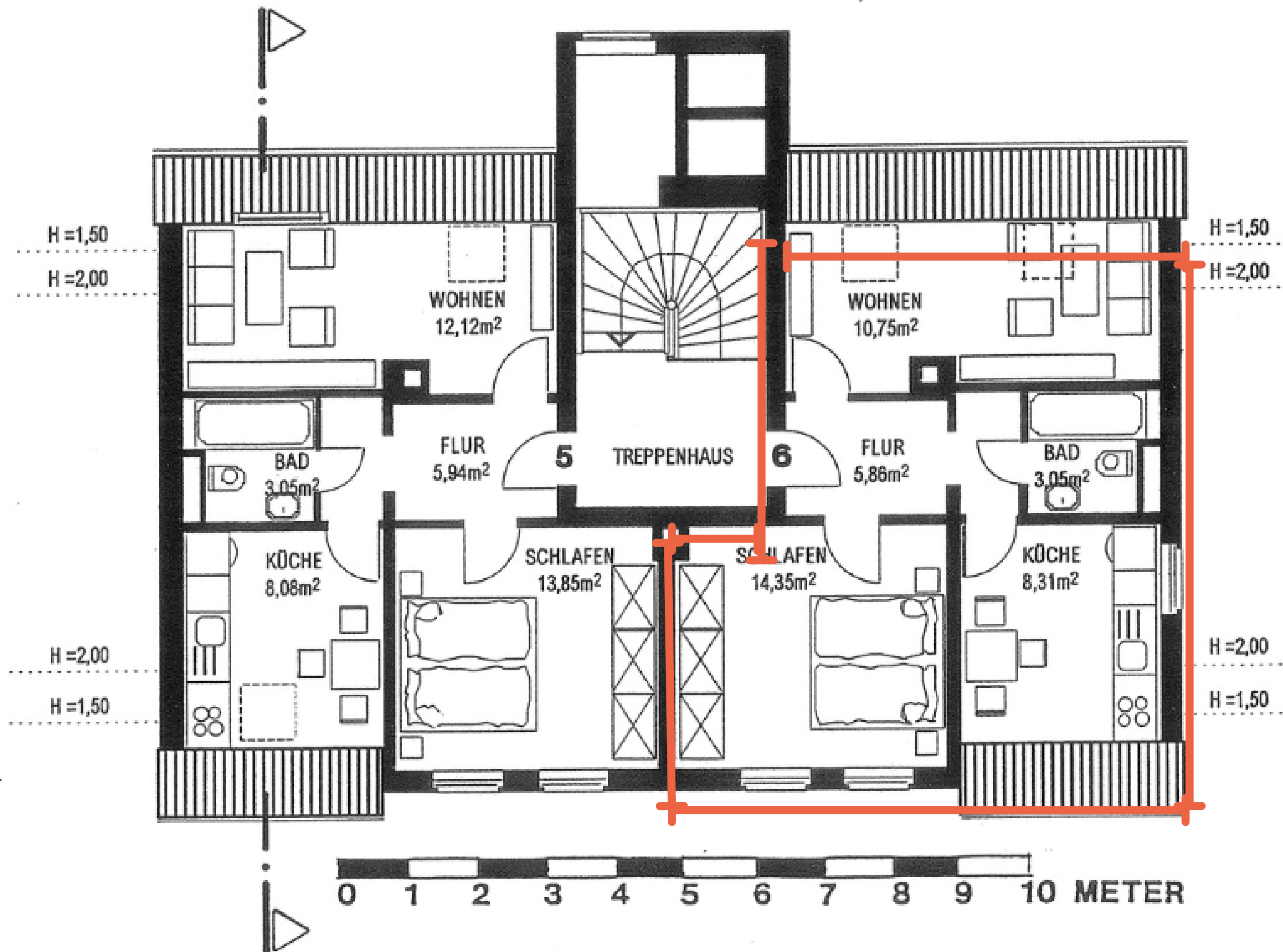
Wohnung 6
