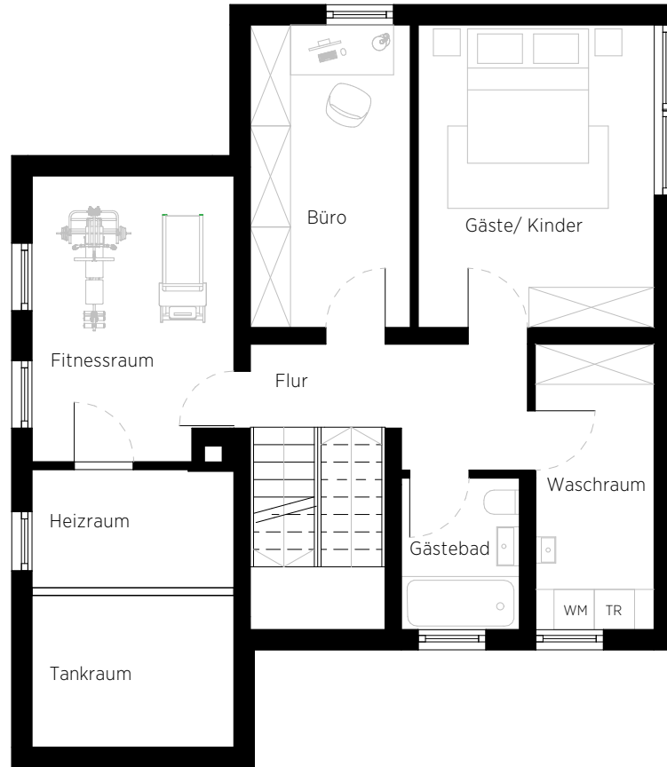
Grundriss UG
